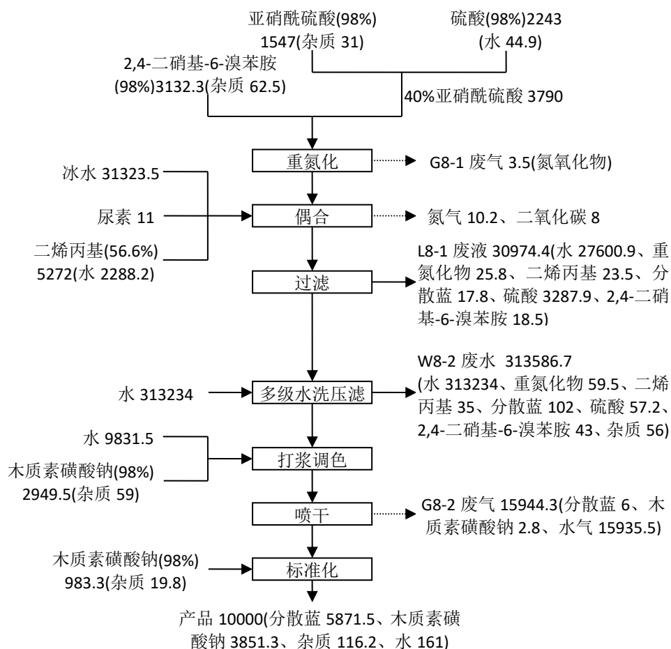
图 4.2-1 分散蓝 291:1#产品生产工艺流程及物料平衡图 (t/a)
