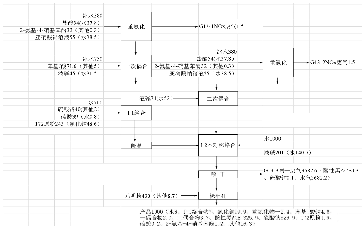
图 4.2-5 酸性黑 ACE 产品生产工艺流程及物料平衡图 (t/a)
