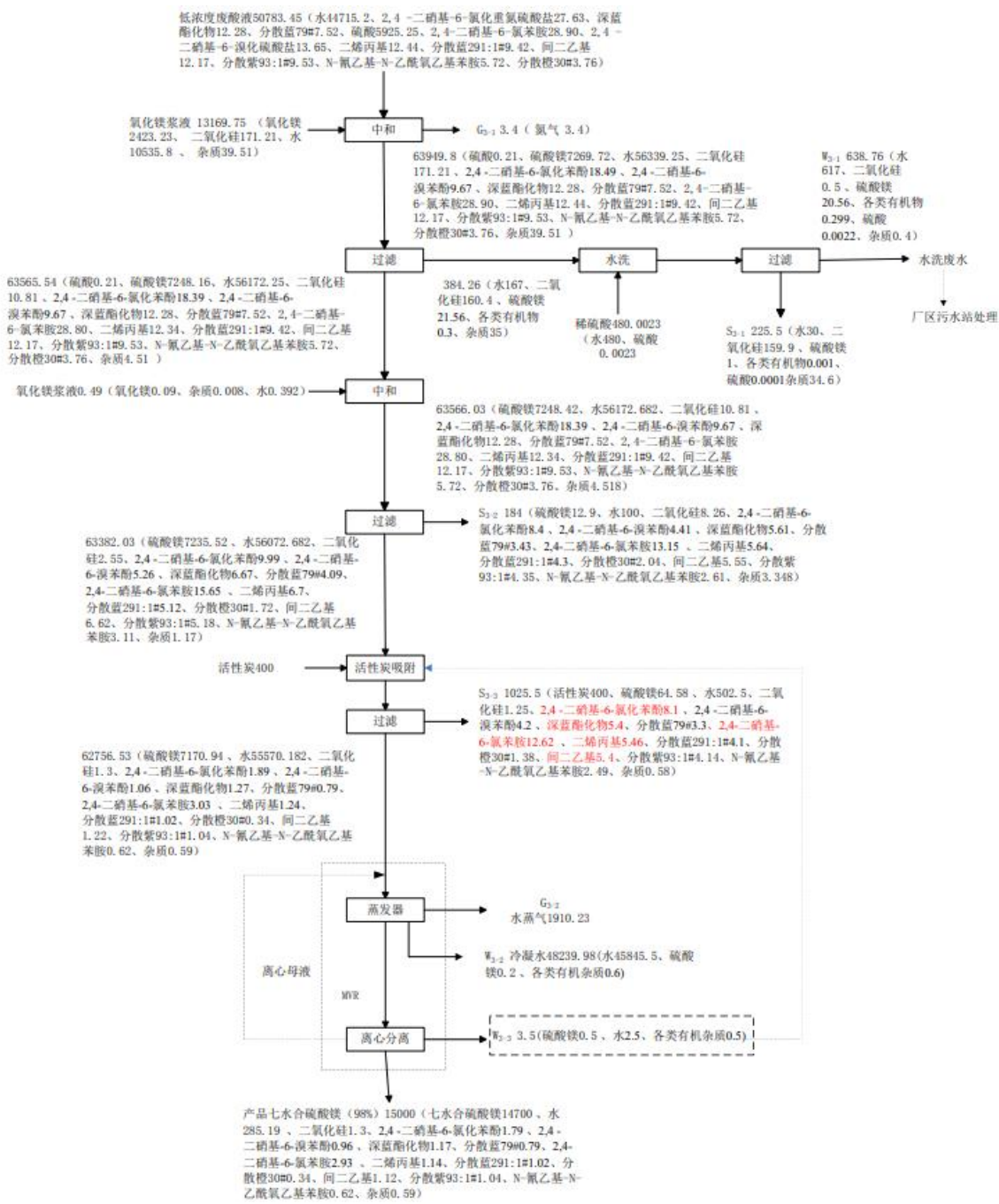
图 4.2-8 七水硫酸镁生产工艺流程图 (t/a)
