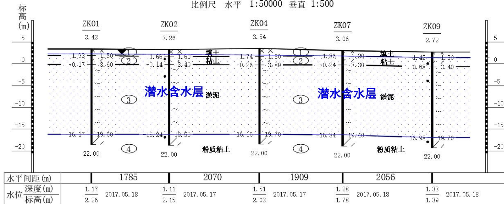
图 3.4-2 水文地质剖面图 (I-I')
