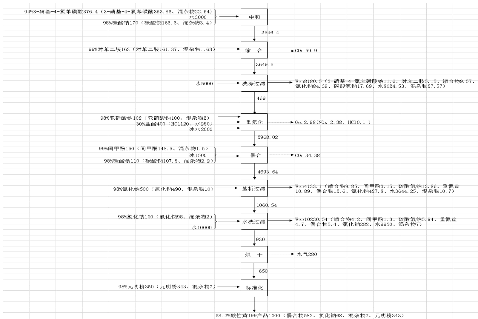
图 4.2-6 酸性黄 199#产品生产工艺流程及物料平衡图 (t/a)
