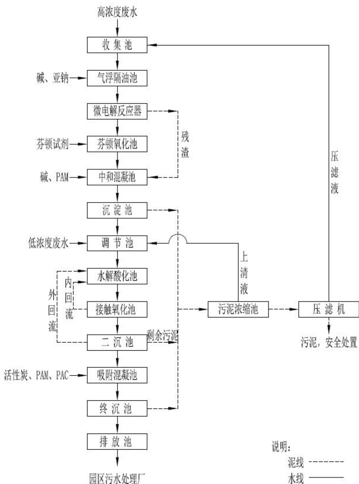
4.3-2 废水处理工艺流程图
