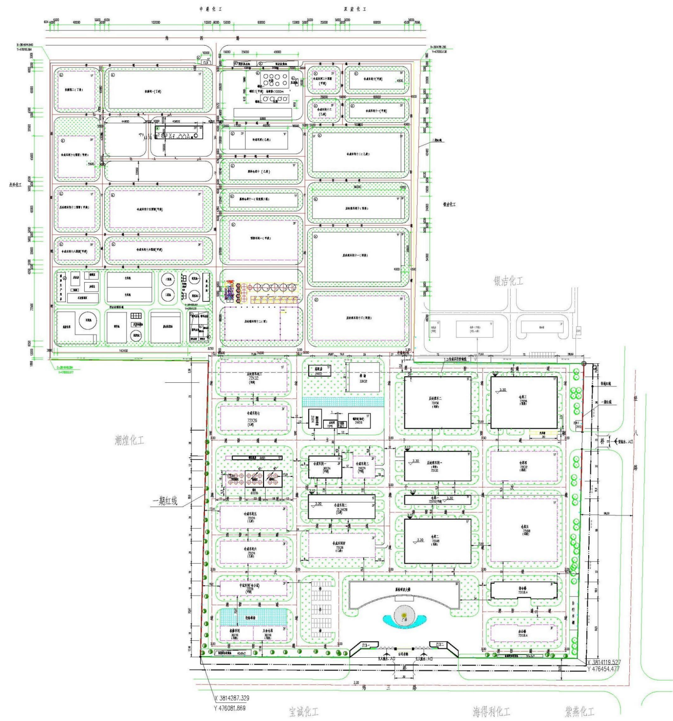
图 4.4-1 边界及平面布置图
