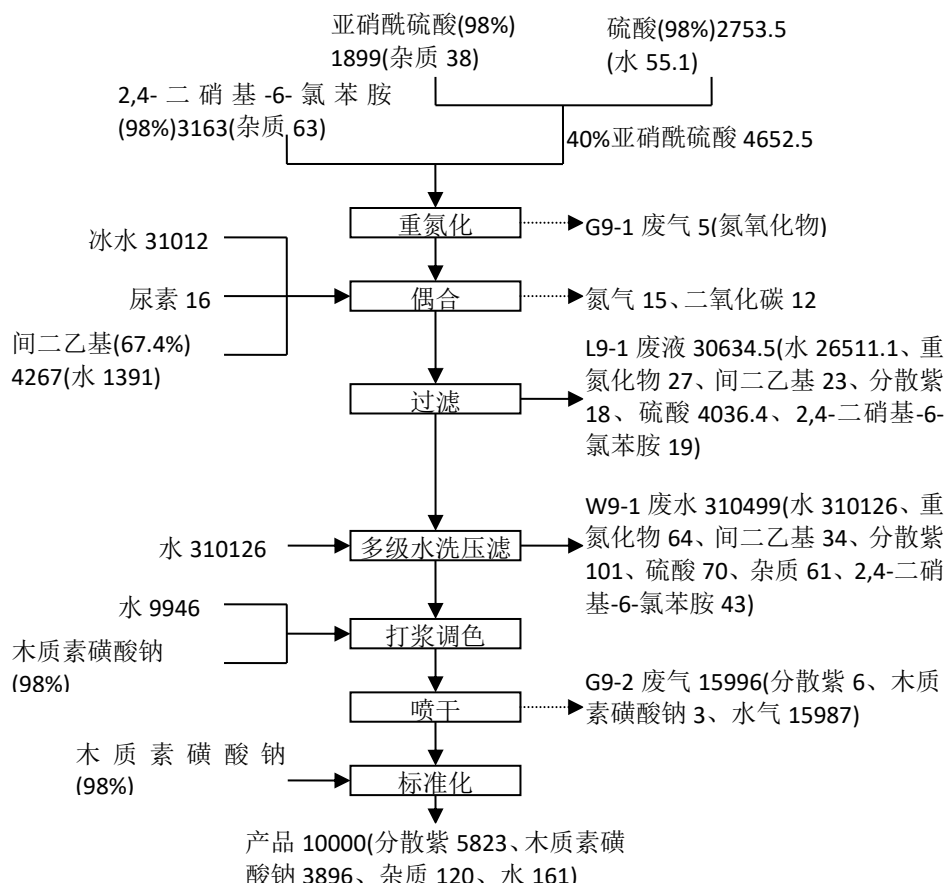
图 4.2-2 分散紫 93:1#产品生产工艺流程及物料平衡图 (t/a)
