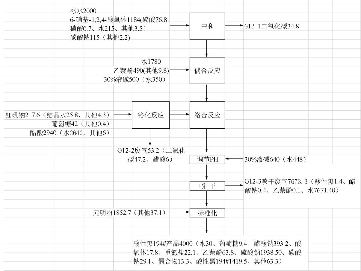
图 4.2-4 酸性黑 194#产品生产工艺流程及物料平衡图 (t/a)
