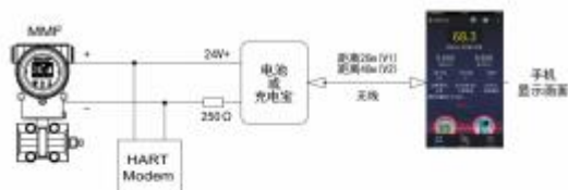
单机运行+外供电接线图 (1)
