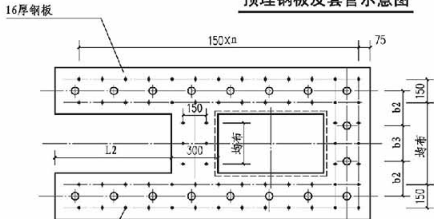
预埋钢板及套管示意图
