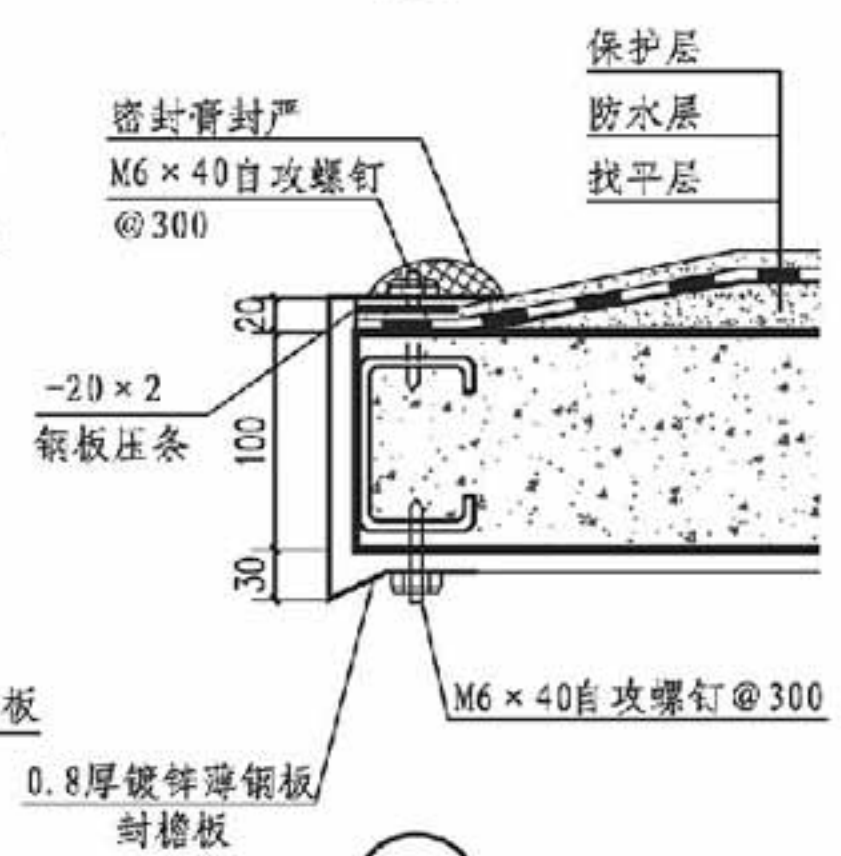
⑤ 板构造
