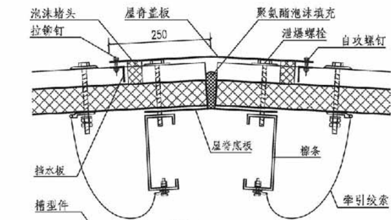
① 双坡屋脊
