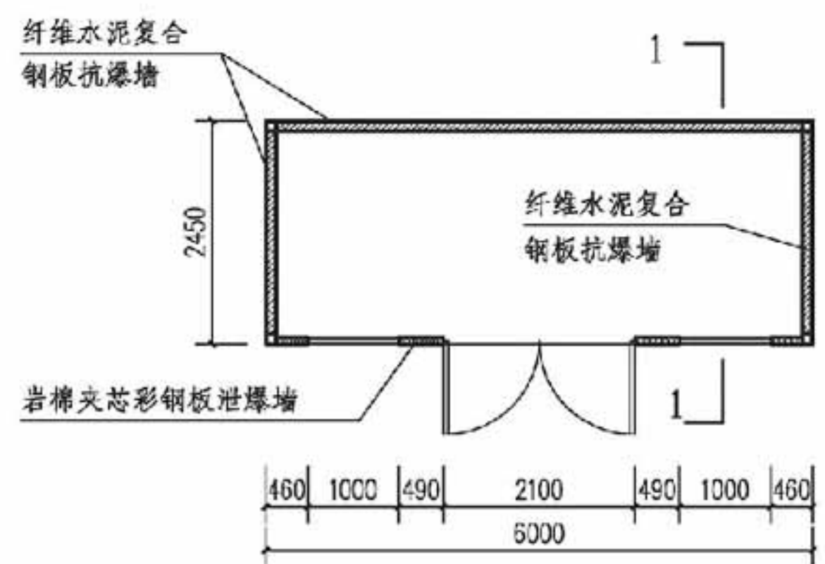
平面图
