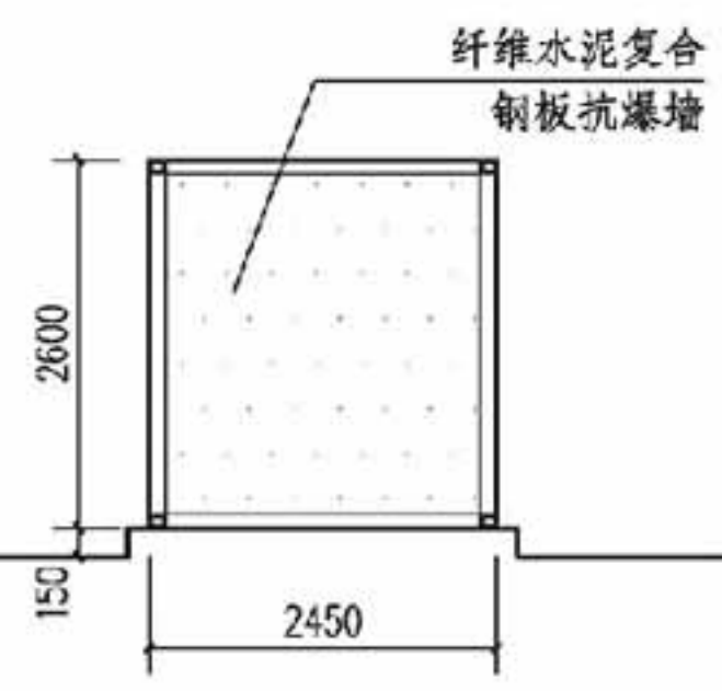
侧立面图
