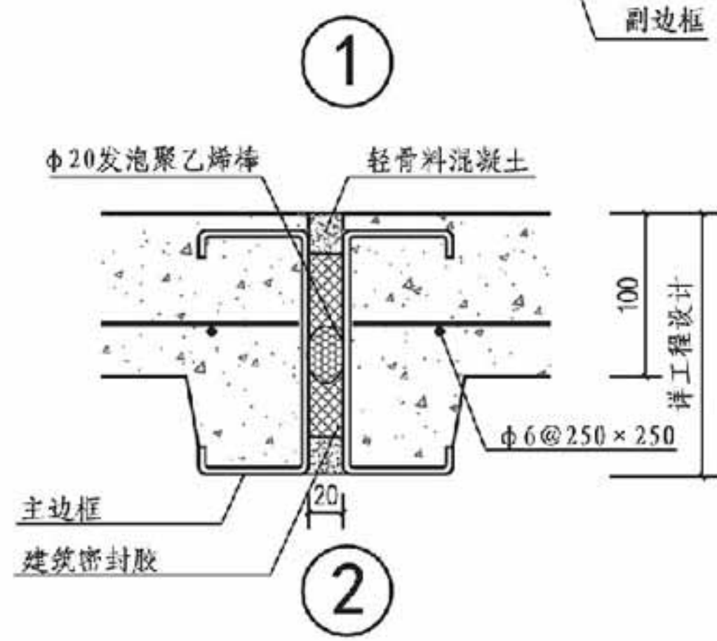
泡沫混凝土复合墙板构造图
