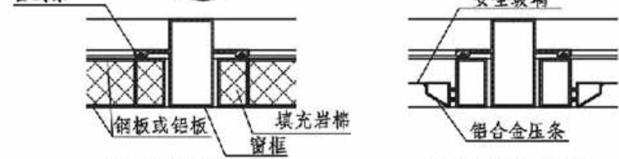
(a) 保温型泄爆窗 (b) 采光型泄爆窗
