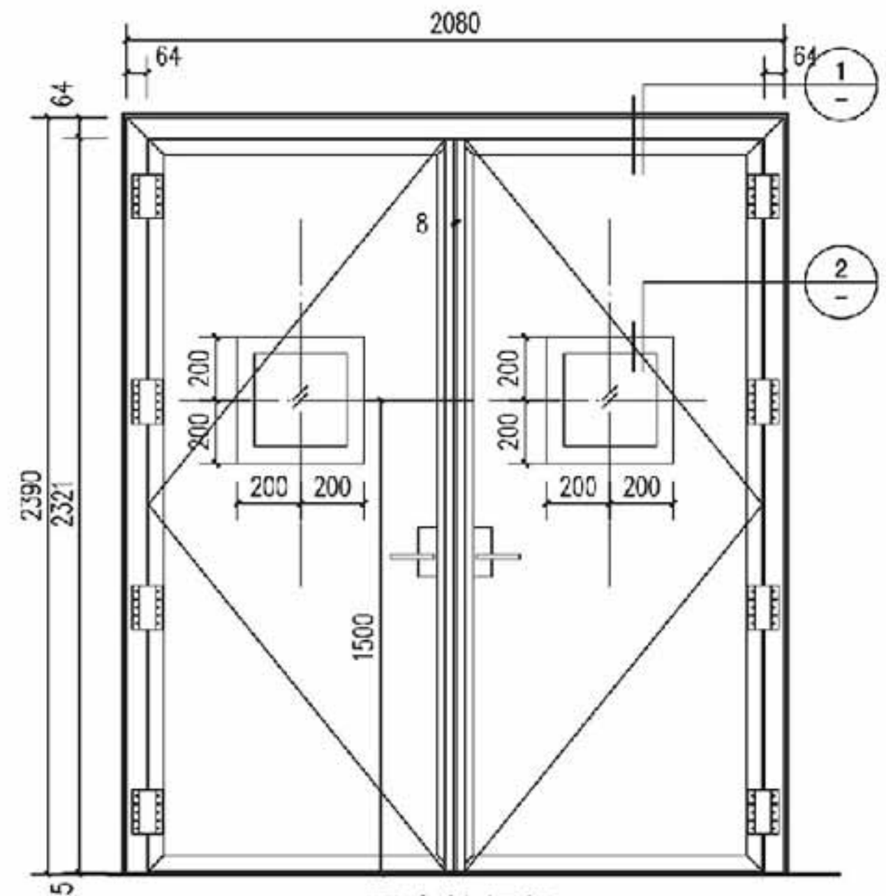
双扇抗爆门 (对称门)
