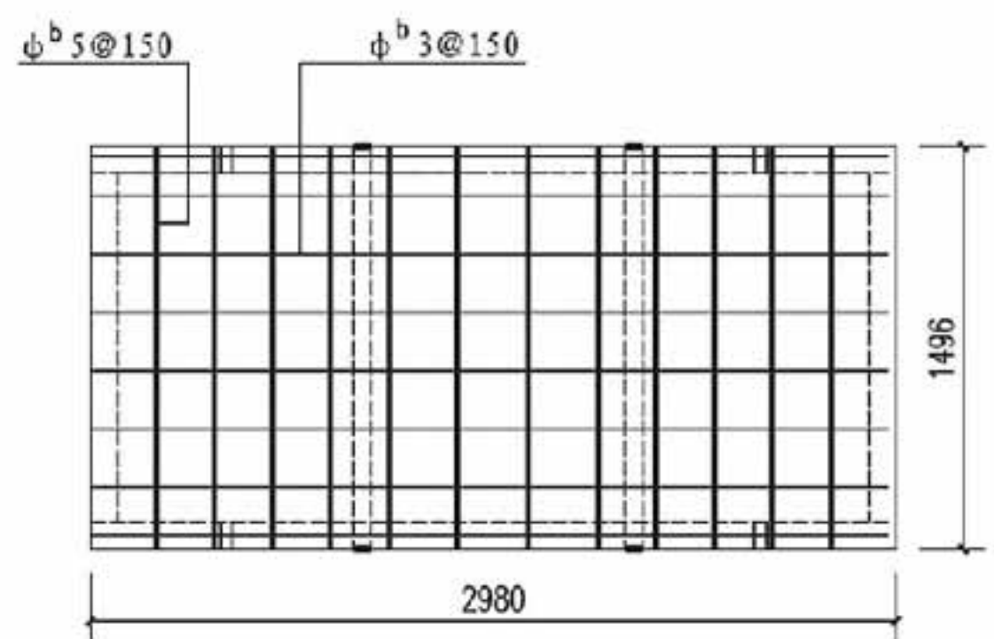
屋面板配筋图
