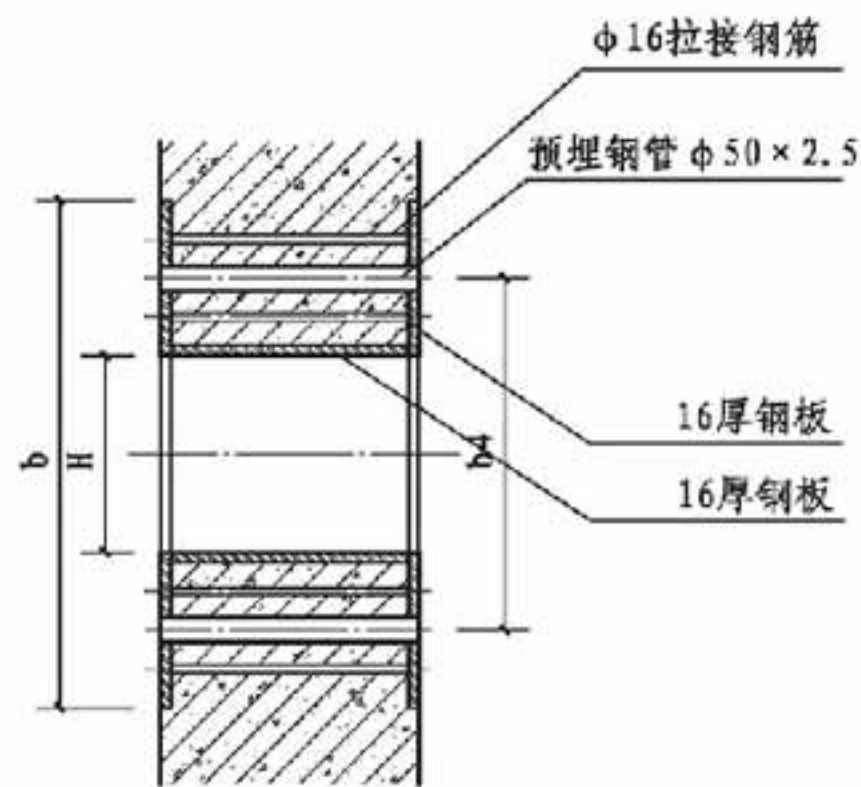
1-1
