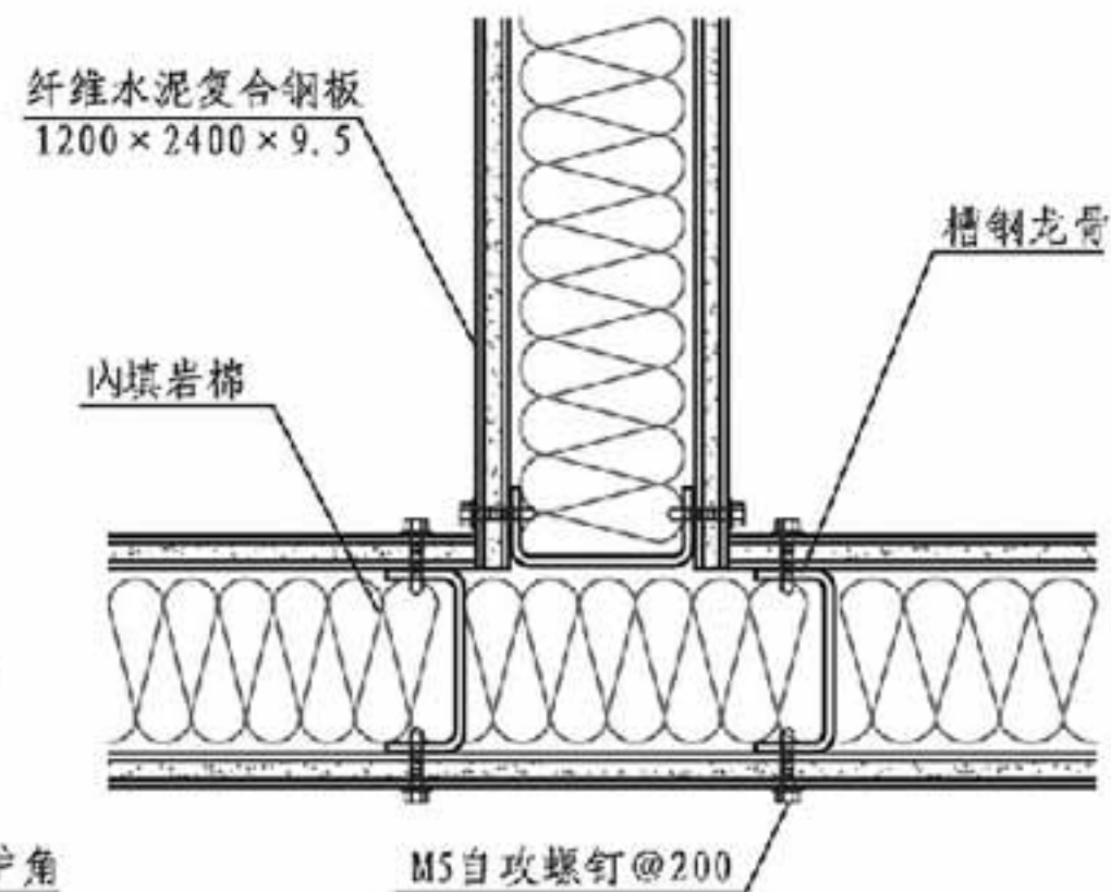
④ 与内墙交接
