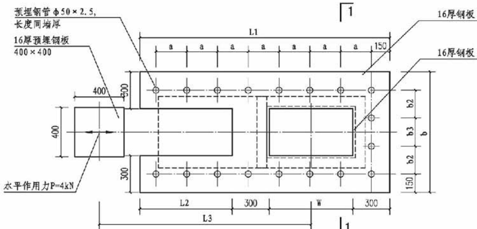
预埋钢板及套管示意图
