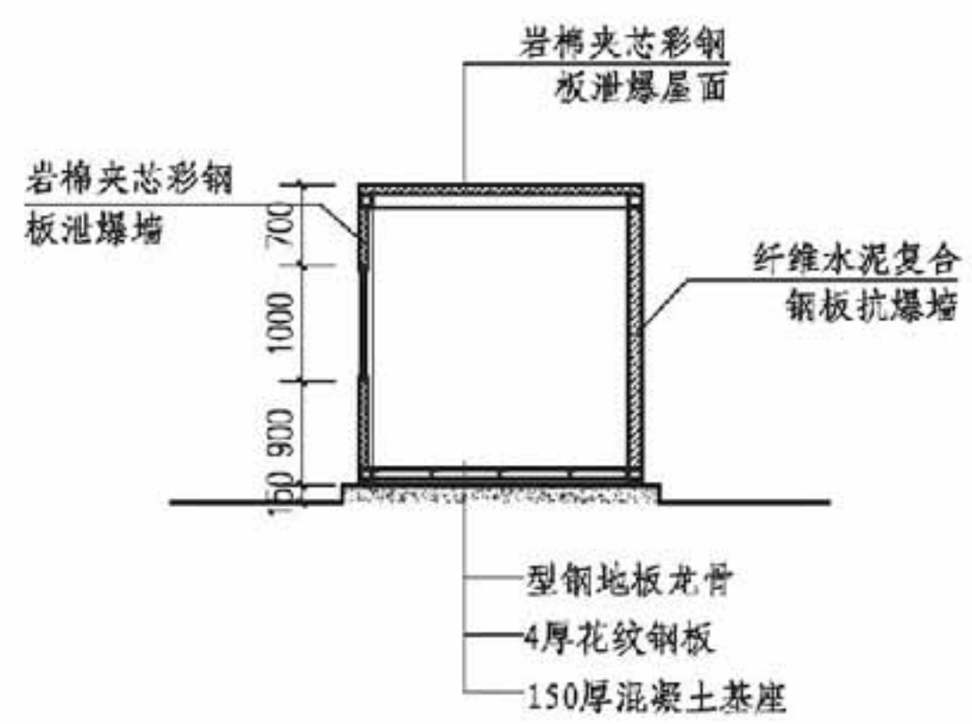
1-1剖面图
