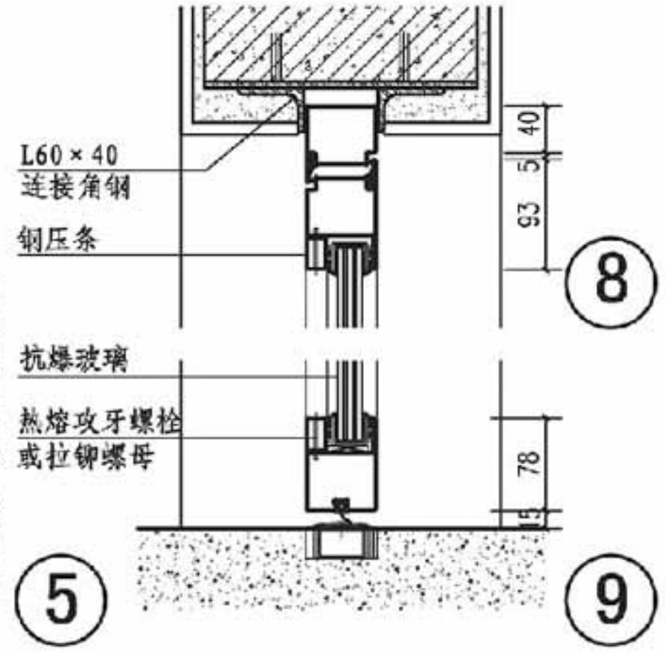
特殊门型玻璃抗爆门详图
