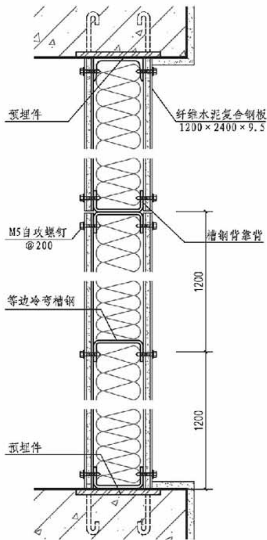
① 与钢筋混凝土梁连接
