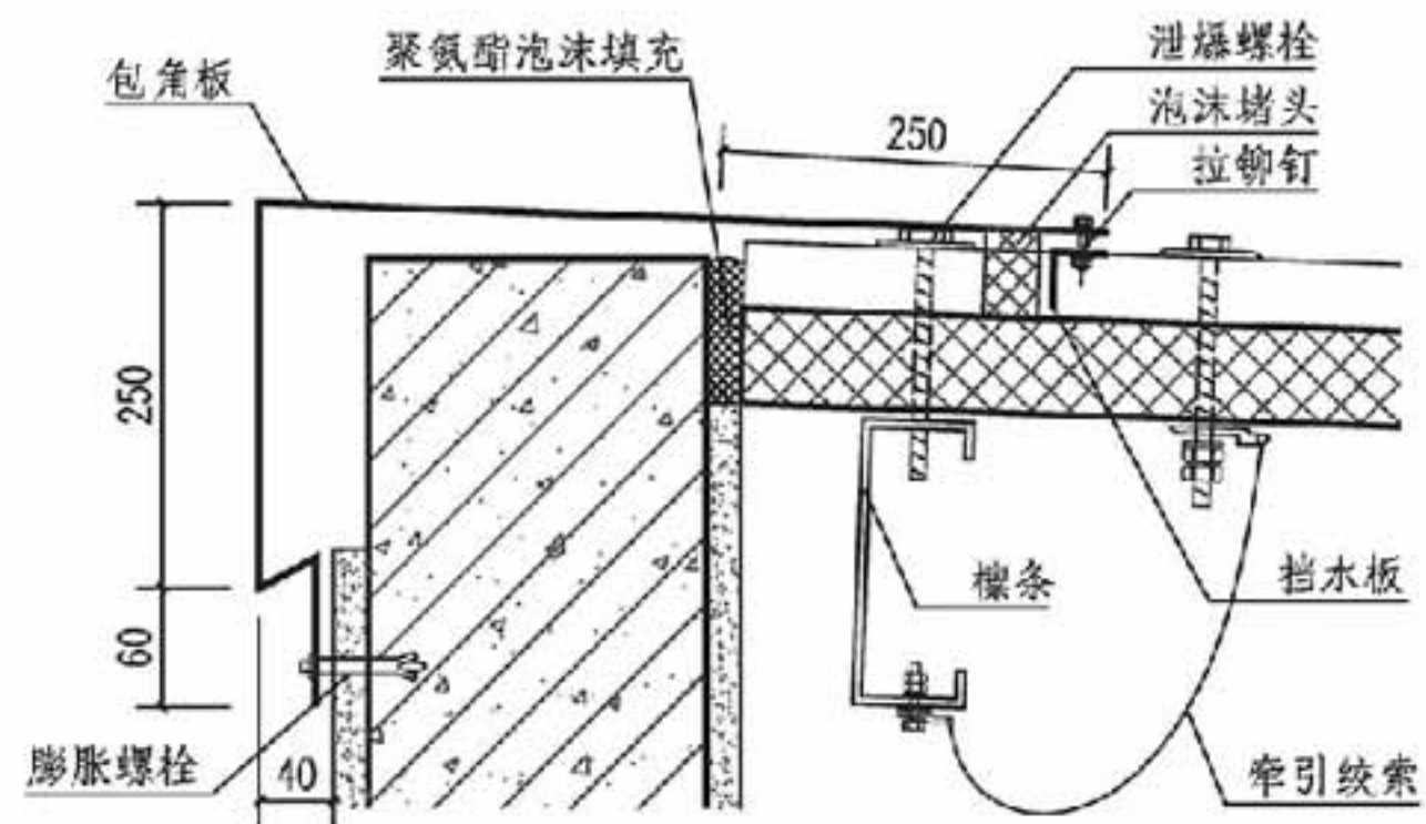
② 单坡屋脊
