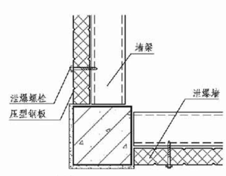
⑥ 内嵌式泄爆墙转角
