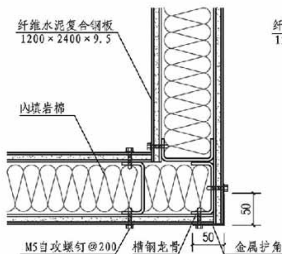
③ 阳角
