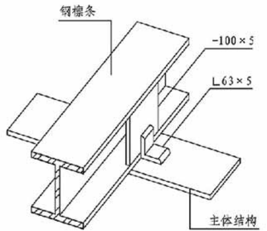
檩条和主体结构连接示意图
