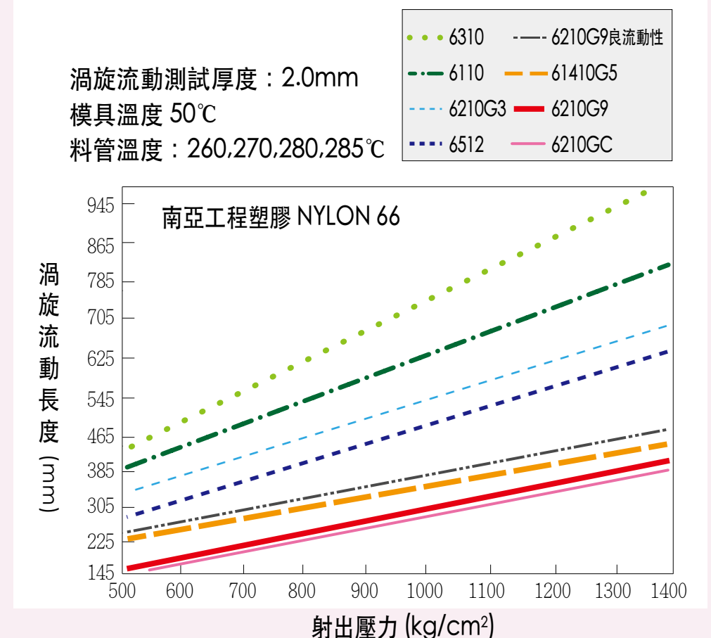
圖 9. 射出壓力對流動長度之影響
