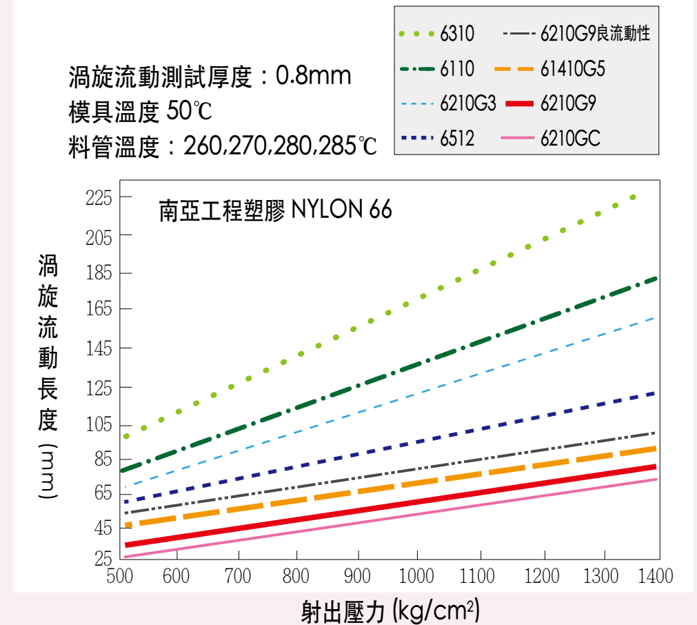
圖 8. 射出壓力對流動長度之影響
