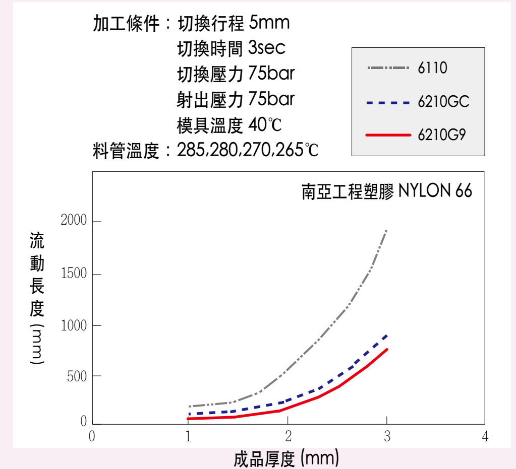
圖 6. 成品厚度對流動長度之影響
