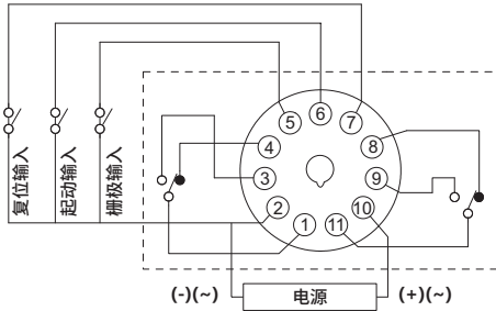
YEDH3BA-N (接点输出)
