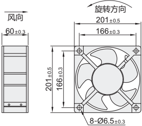
外形尺寸: 20060M2
