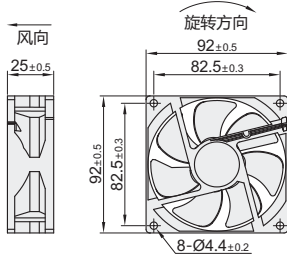
外形尺寸: 92/9225L2
