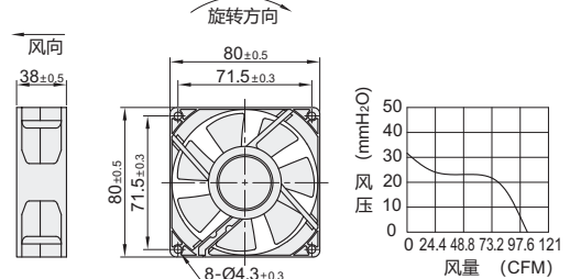
外形尺寸: 8038H2
