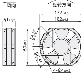
外形尺寸: 17251M2
