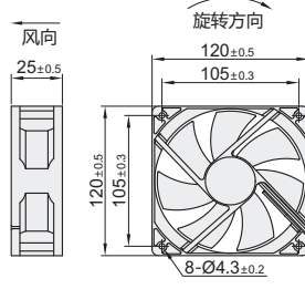
外形尺寸: 120B
