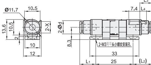
小型真空过滤器 YEDJ-WEX11
