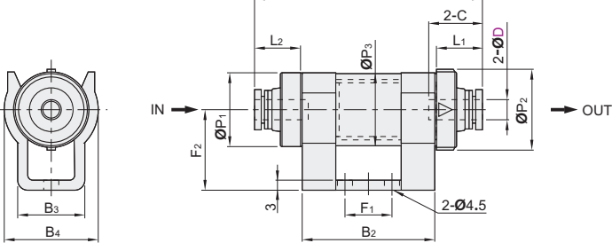
标准型真空过滤器 YEDJ-WEX31
