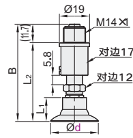
弹簧式直接安装型 YEDJ-WET76/77
