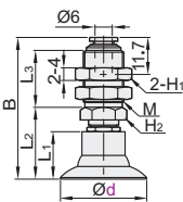
弹簧式侧面真空端口 YEDJ-WET71/72
