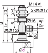
弹簧式侧面真空端口 YEDJ-WET71/72
