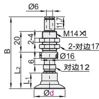
弹簧式顶部真空端口 YEDJ-WET66/67
