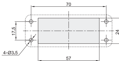
面板开孔图
