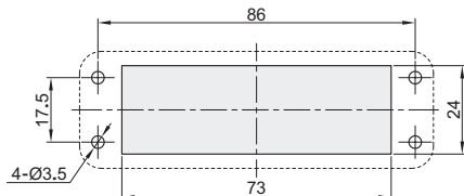
面板开孔图
