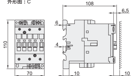
外形图 : C
