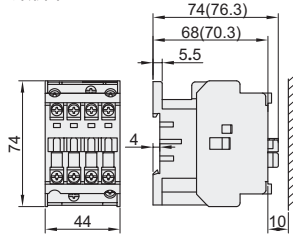
外形图 : A
