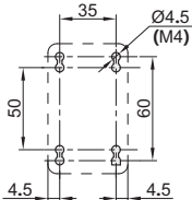
外形图 : A
