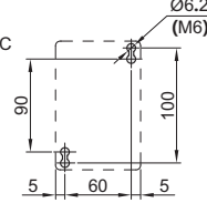
外形图 : C
