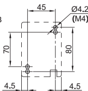
外形图 : B
