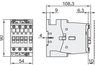
外形图 : B
