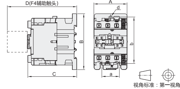
外形图:B
