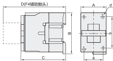
外形图:A
