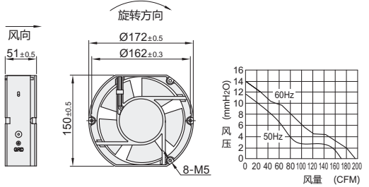
外形尺寸: 172
