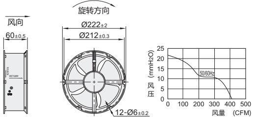
外形尺寸: 220
