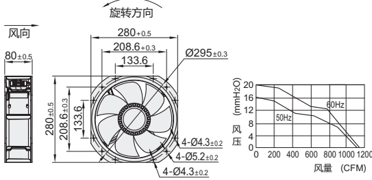
外形尺寸: 280
