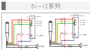
◎接线方式(Connect type)：C, 触点式(Contact type)
