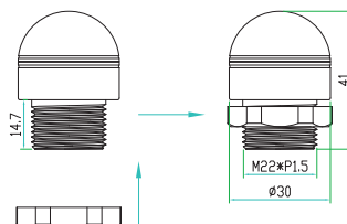
直接出线
