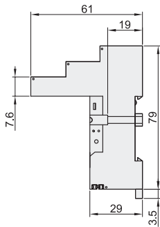
YEDRXZE2S通用侧视图
