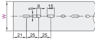
W ≤ 70mm 线槽底部孔尺寸
