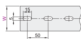
W ≤ 70mm 线槽底部孔尺寸
