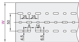
□ W≥70mm线槽底部尺寸
