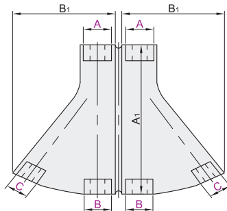
展开视图
