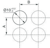
E10安装尺寸 / E10 Installation size
