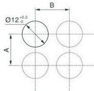
E12安装尺寸 / E12 Installation size
