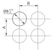
E12安装尺寸 / E12 Installation size
