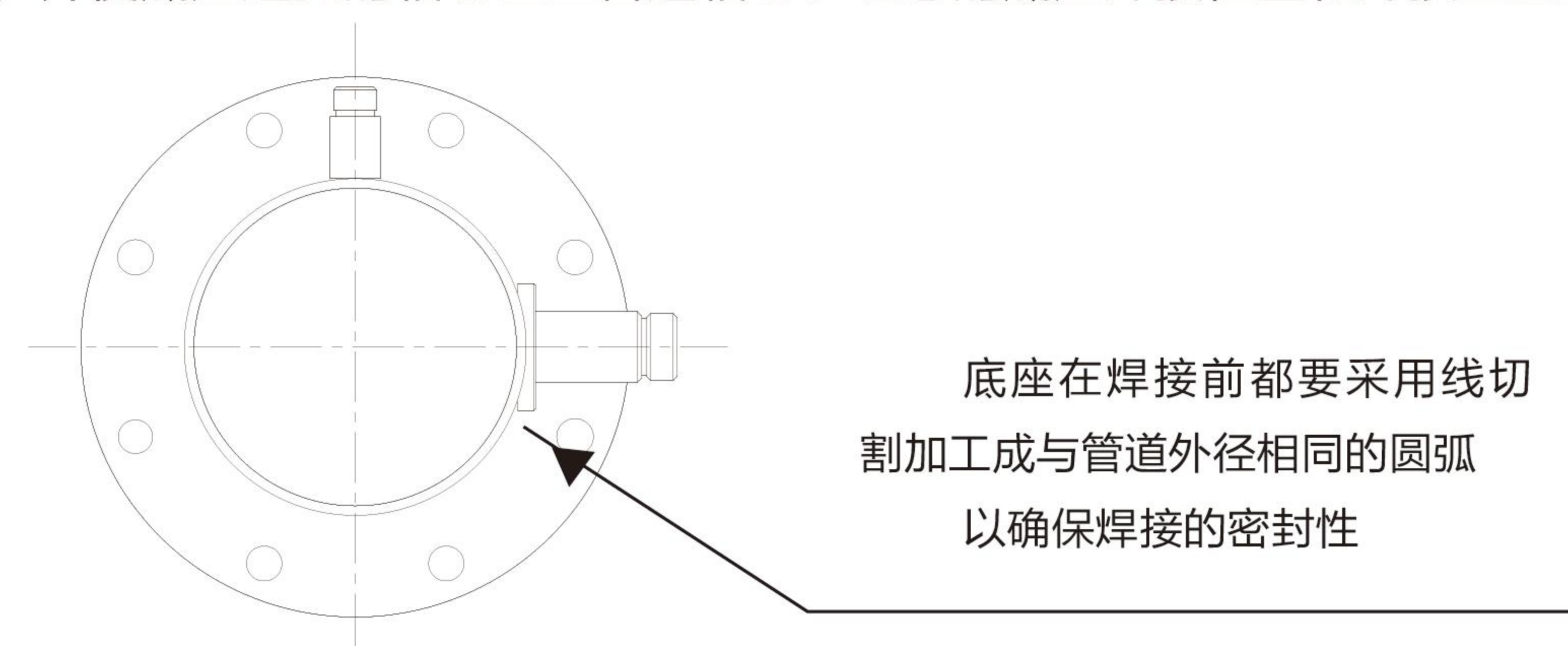
图 7 理想底座焊接位置
