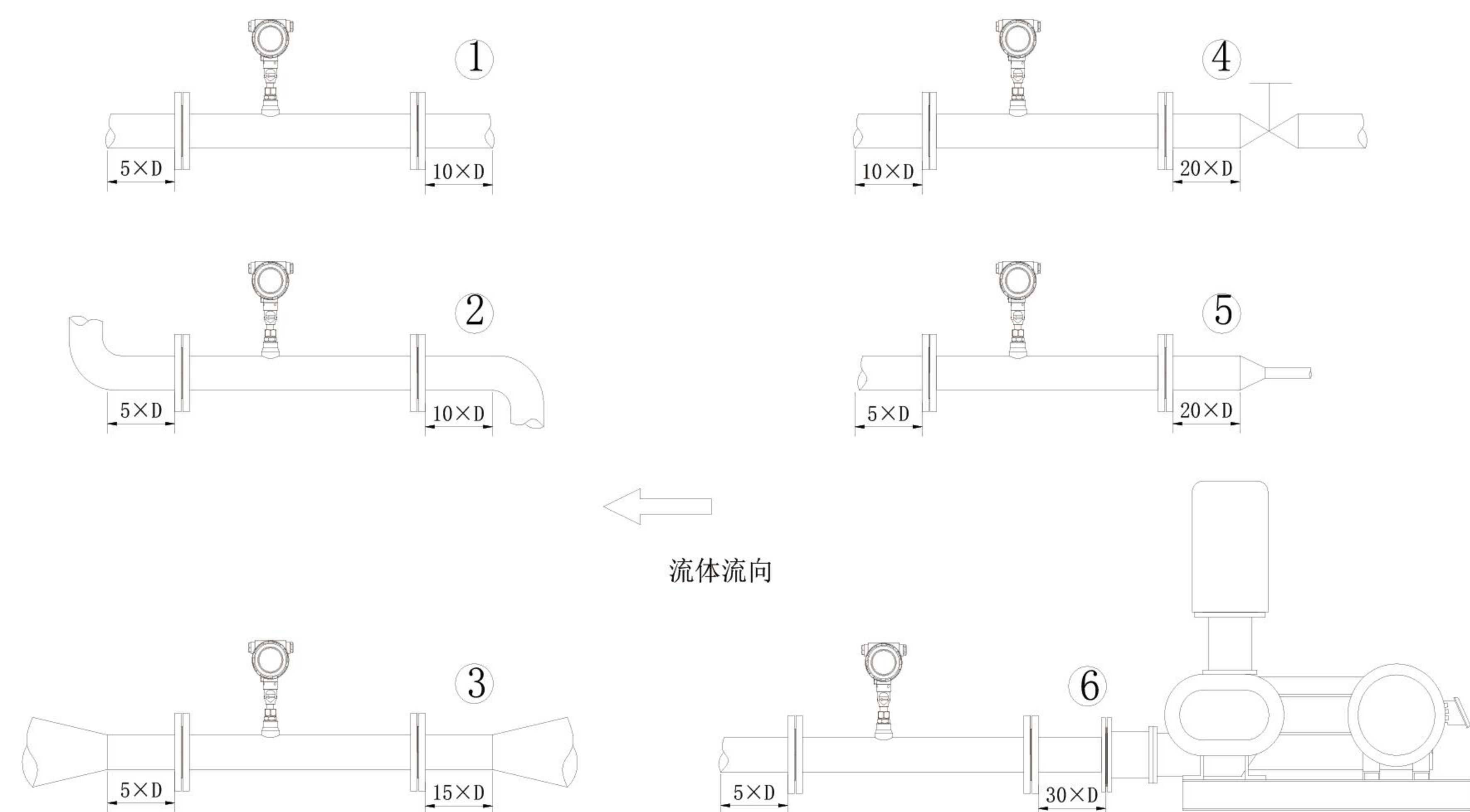
安装前后直管段图
