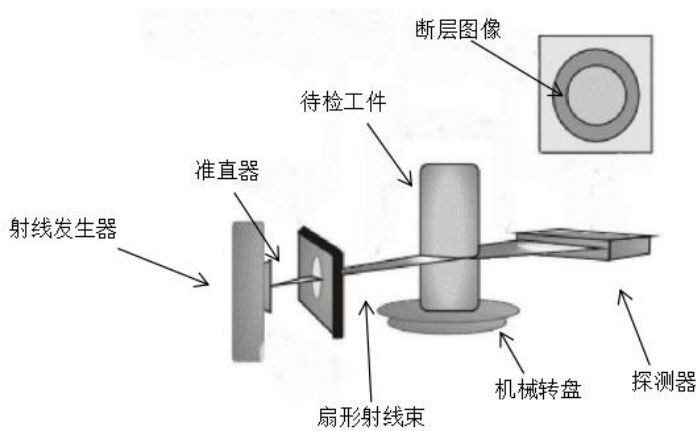
图 9-2 X 射线管线及 X 射线产生的示意图
