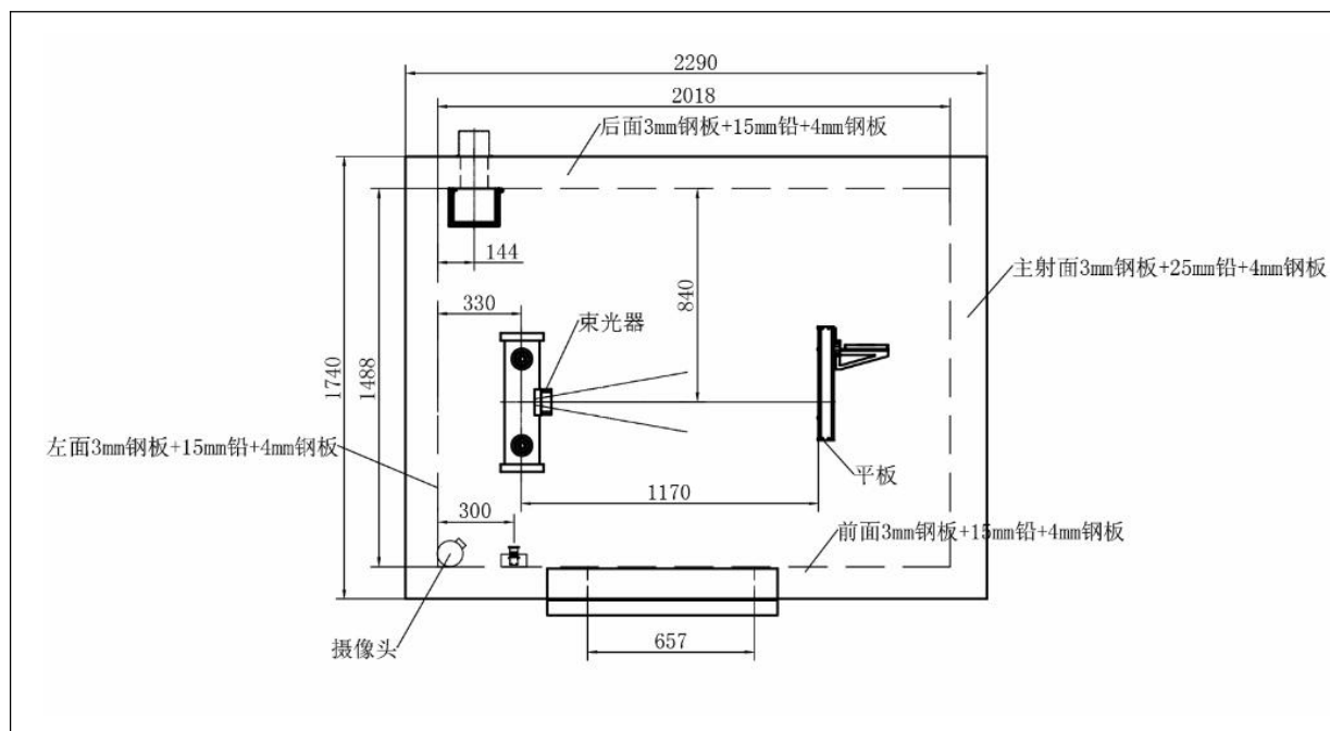
图 10-2 X 射线数字成像检测设备防护设计图 (2)
