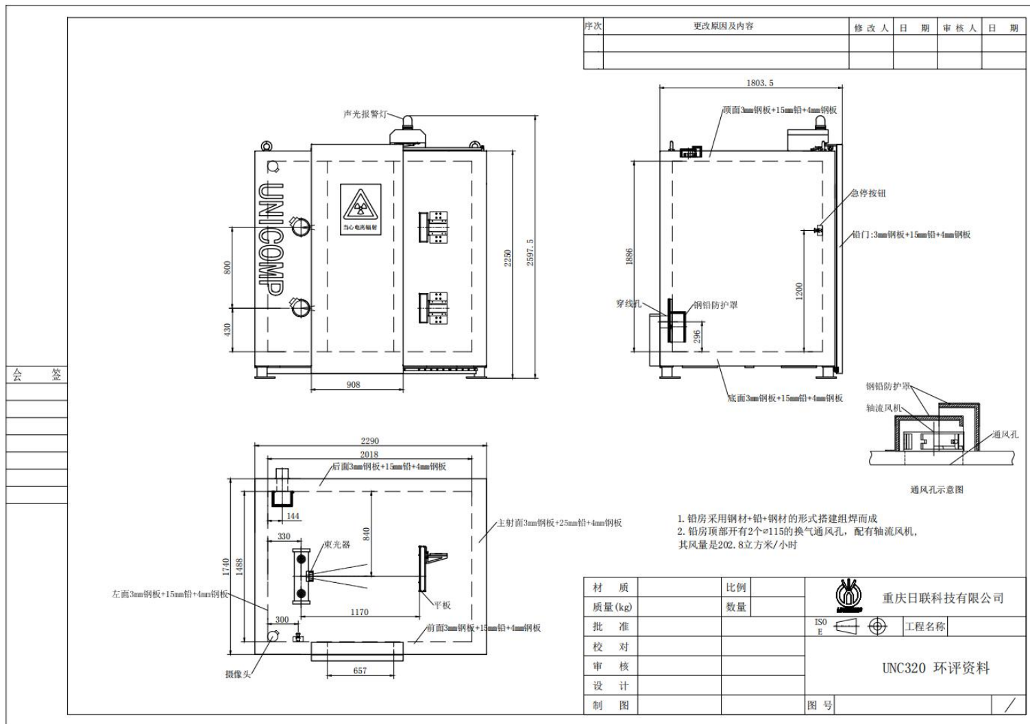
附图 2 设备辐射防护设计图
