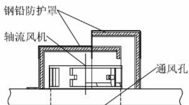
通风孔示意图
