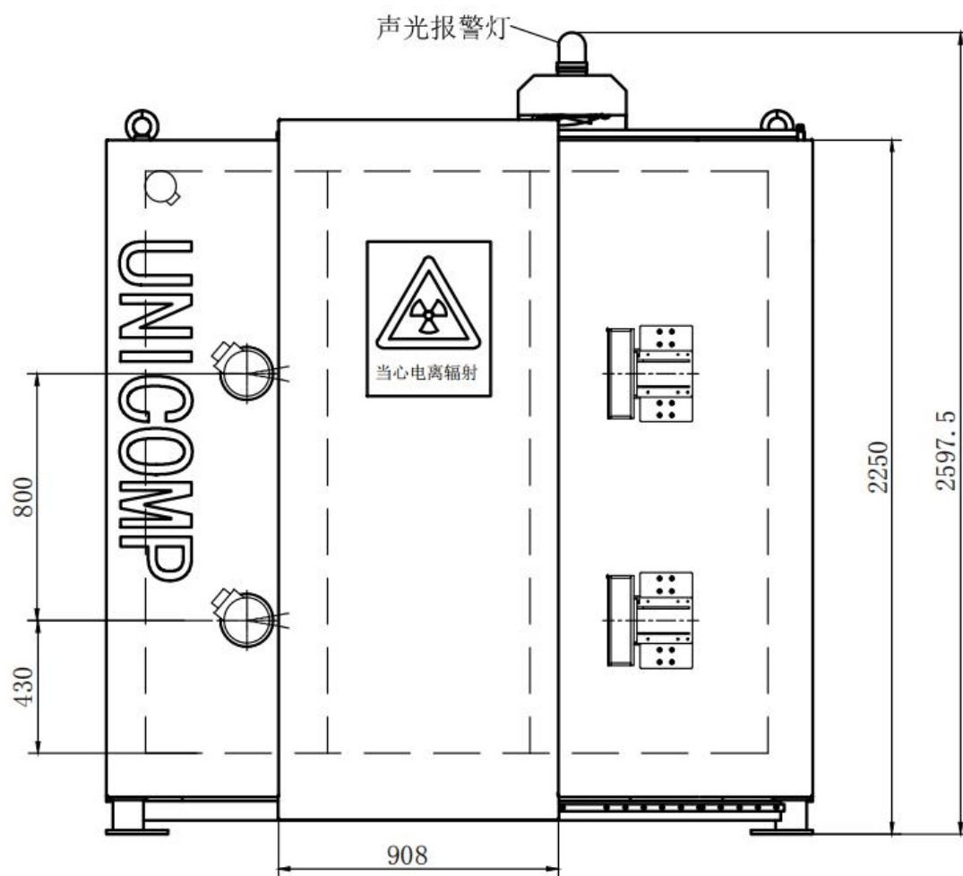
图 10-3 X 射线数字成像检测设备防护设计图 (2)
