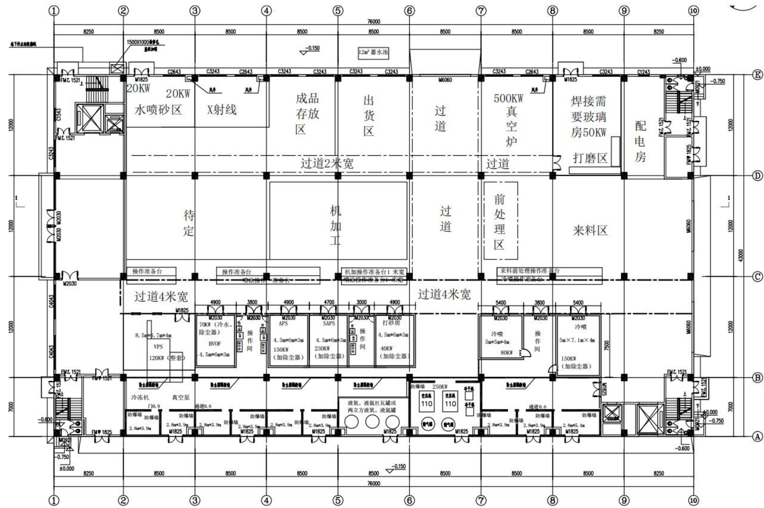
附图 1 车间一首层平面布局图
