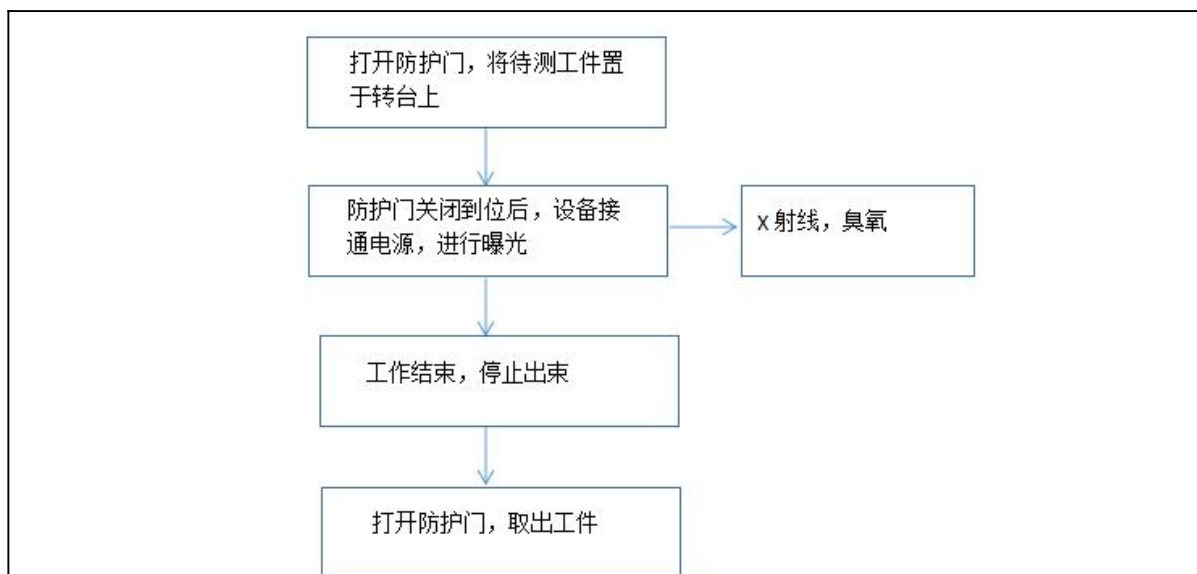
图 9-4 X 射线数字成像检测设备操作流程及产污环节示意图
