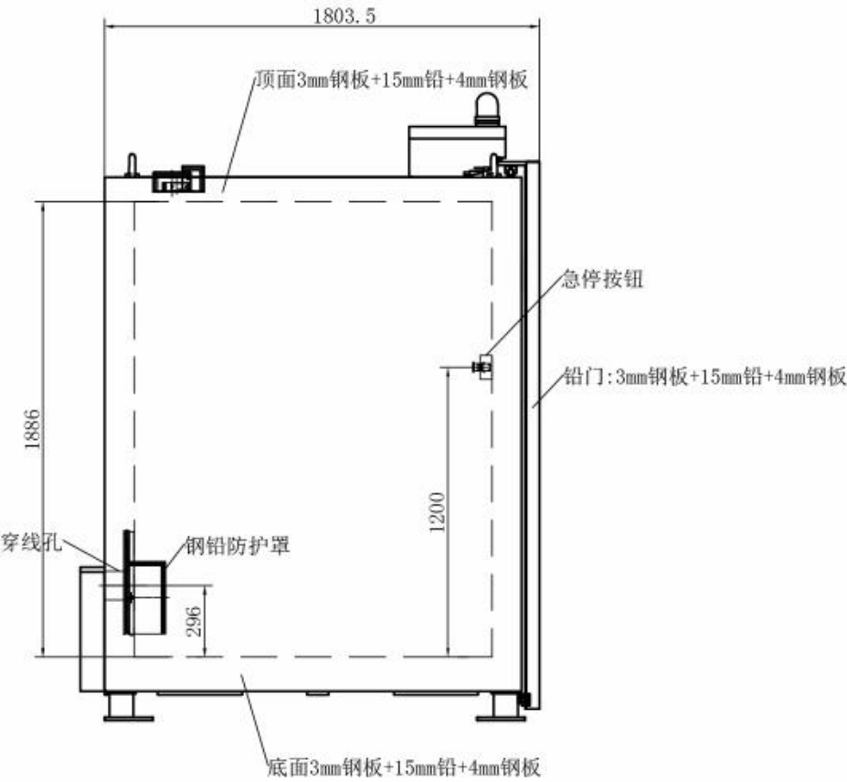
图 10-1 X 射线数字成像检测设备防护设计图（1）
