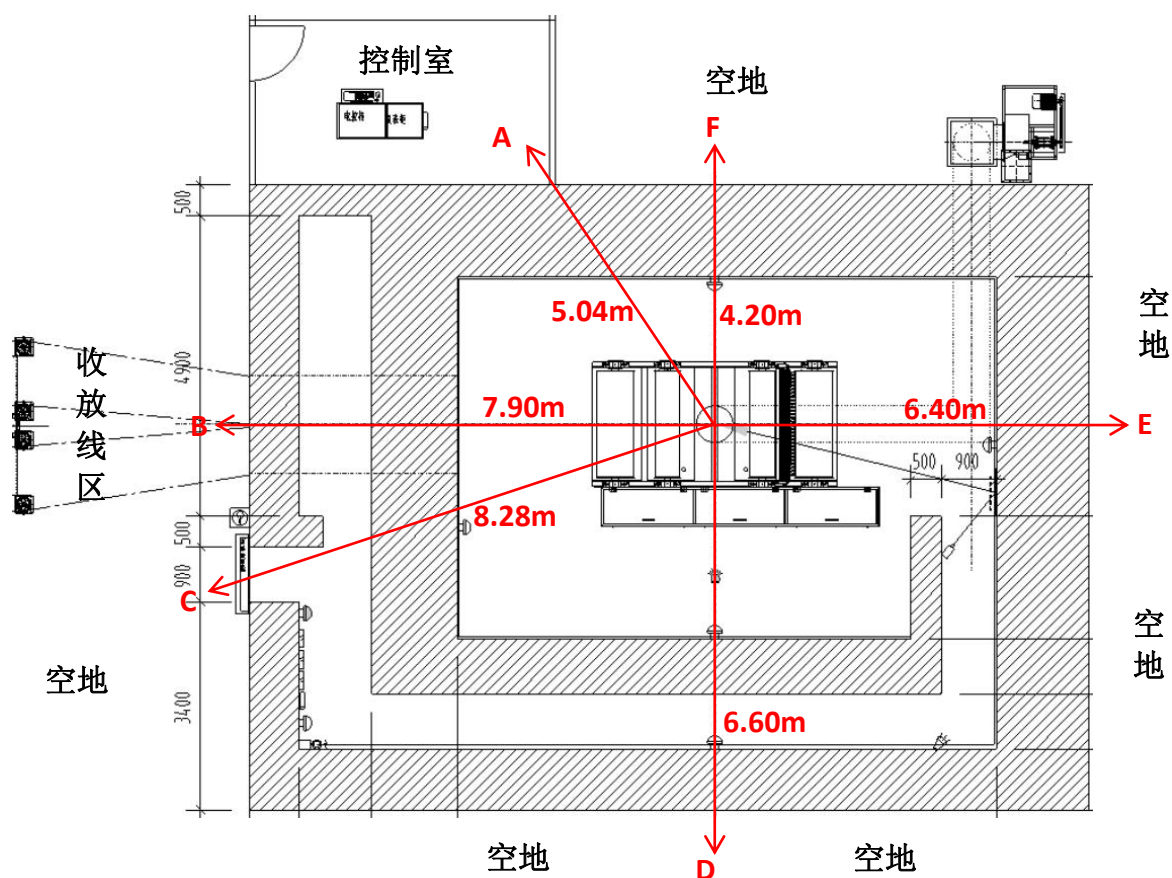
图 11-2 辐照室平面目标关注点
