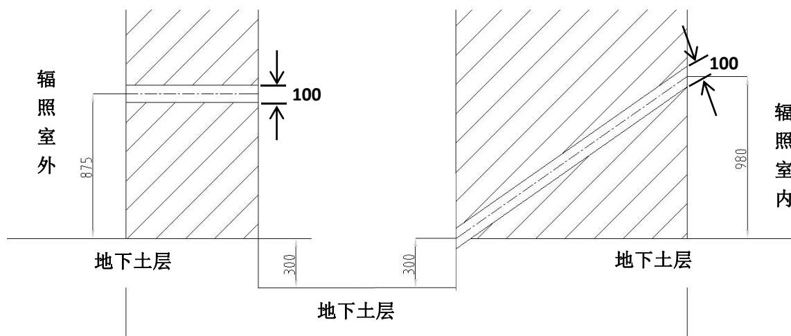
图 10-5 图 10-4 中虚线圆圈部分放大图
