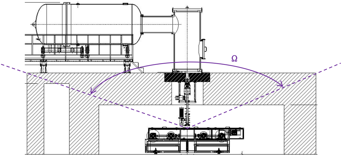
图 11-4 立体角计算示意图
