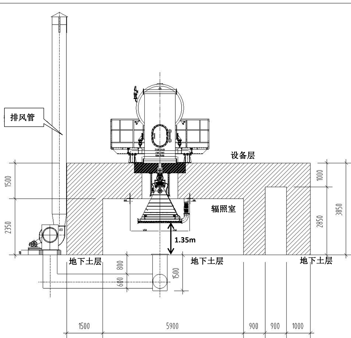
图 10-3 辐照室西南-东北方向剖面设计图
