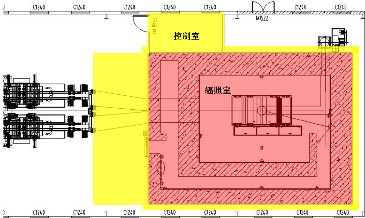
图 10-15 辐照室工作场所分区图（红色为控制区，黄色为监督区）
