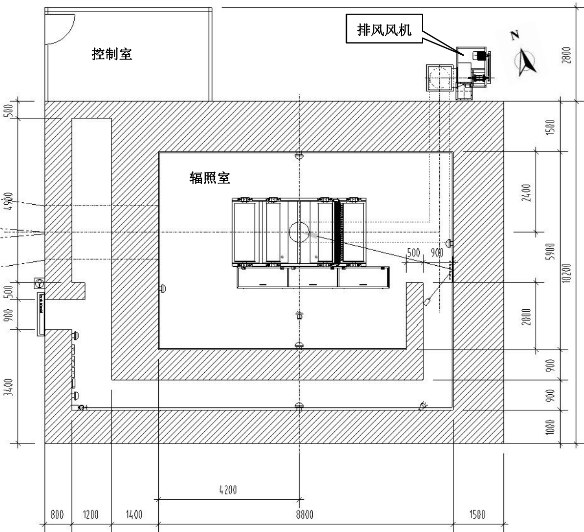
图 10-1 辐照室平面设计图
