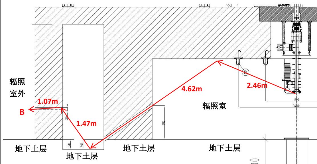
图 11-5 辐照室的辐照材料进出孔的散射路径
