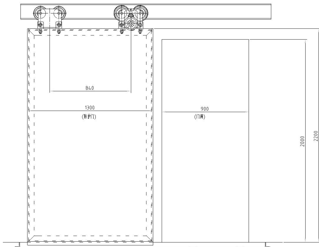
图 10-7 辐照室防护门设计图
