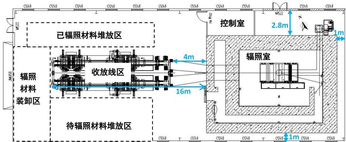
图 1-4 辐照车间平面布局图
