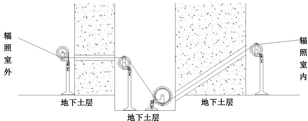
图 10-6 辐照材料进出辐照室示意图
