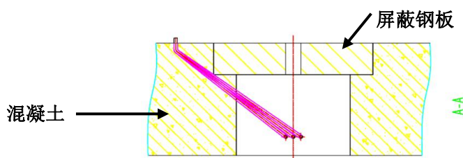
图 10-10-1 电缆沟穿过屏蔽墙的设计图（剖面图）
