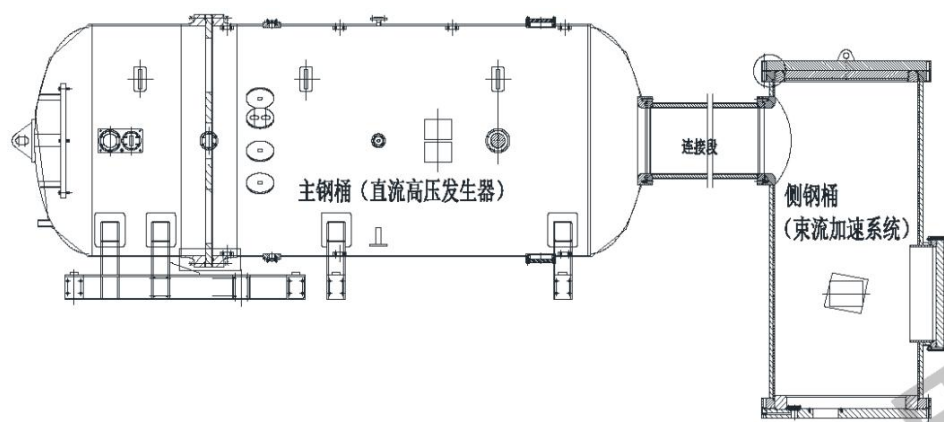
图 9-3 DDLH2.0/50-1600 型电子加速器主体装置示意图
