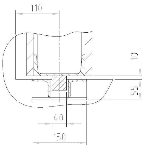
图 10-8 辐照室防护门底部安装剖面设计图
