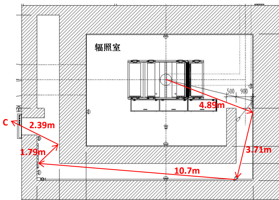
图 11-3 辐照室迷路散射路径
