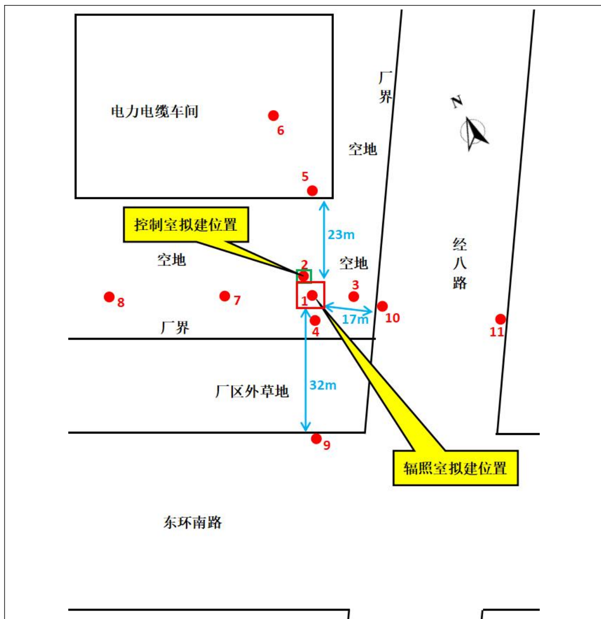
图 8-2 检测布点图
