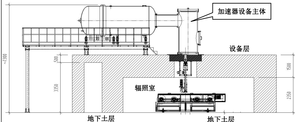
图 9-4 DDLH2.0/50-1600 型电子加速器整体结构示意图
