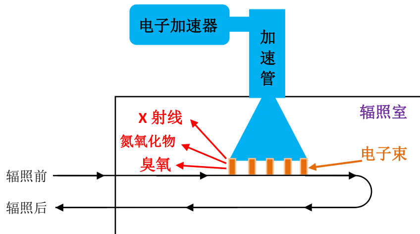
图 9-5 使用电子加速器的电子束进行辐照交联的主要产污环节示意图
