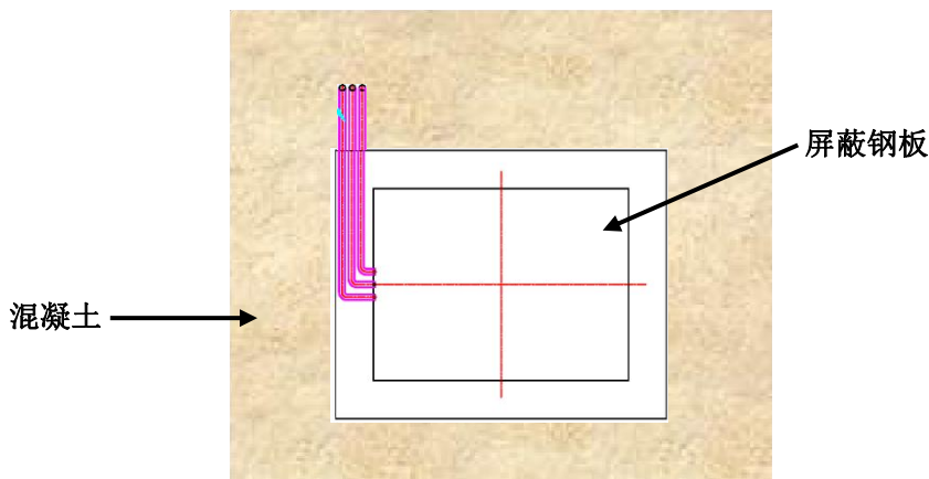
图 10-10-2 电缆沟穿过屏蔽墙的设计图（俯视图）
