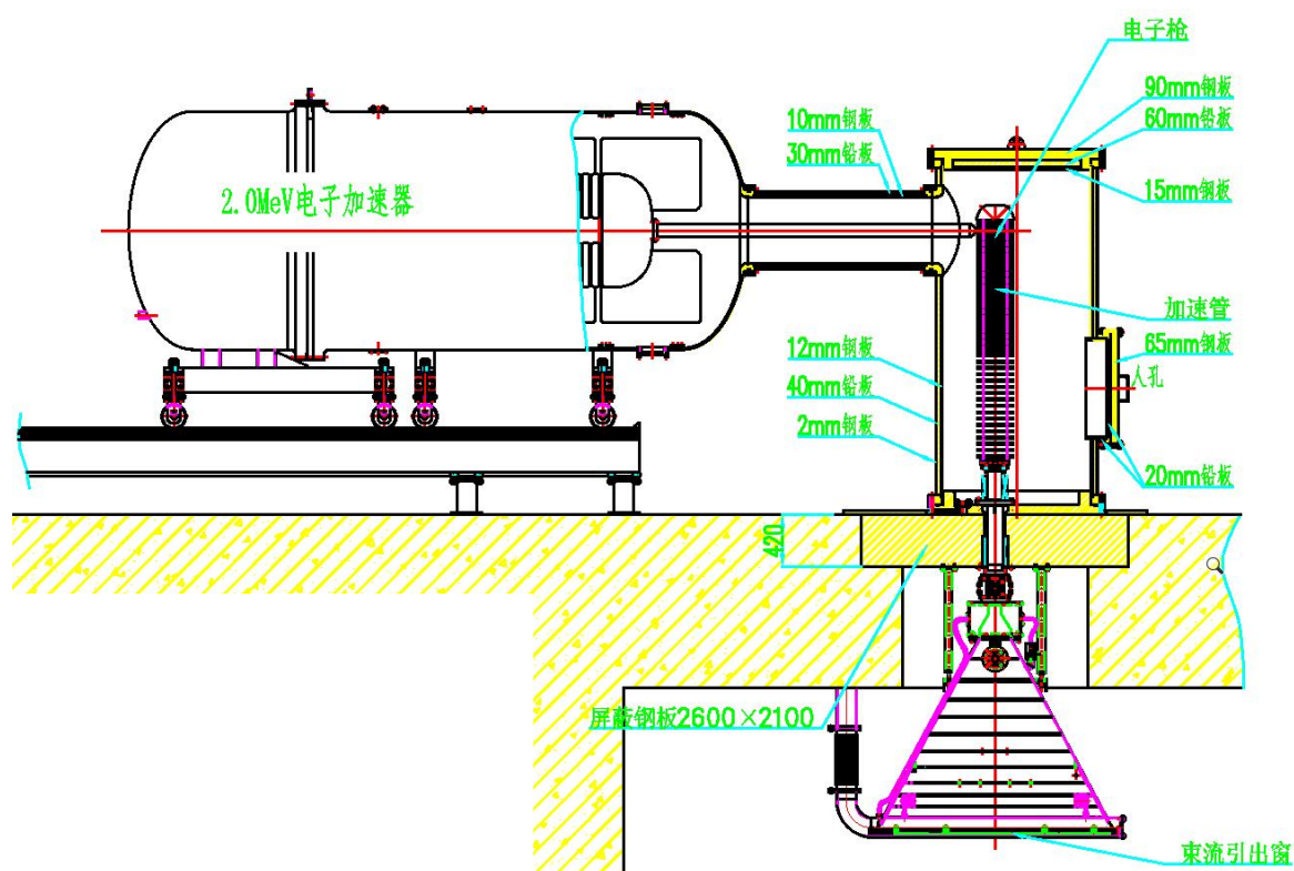
图 10-9 DDLH2.0/50-1600 型电子加速器设备本身自带的辐射屏蔽设施
