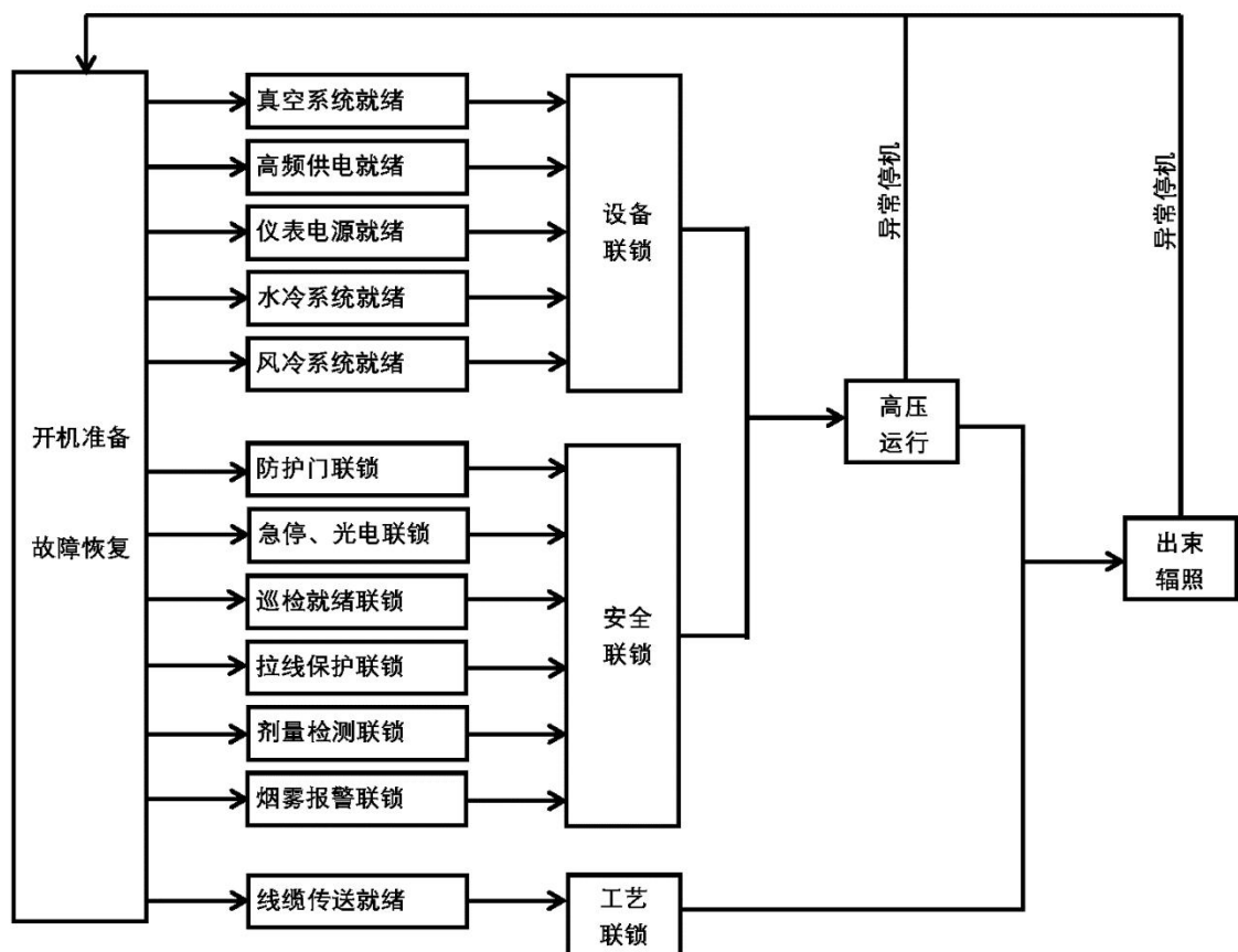
图 10-14 设备安全联锁图
