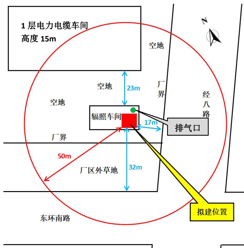
图 10-12 辐照室排风系统的排风口平面位置图
