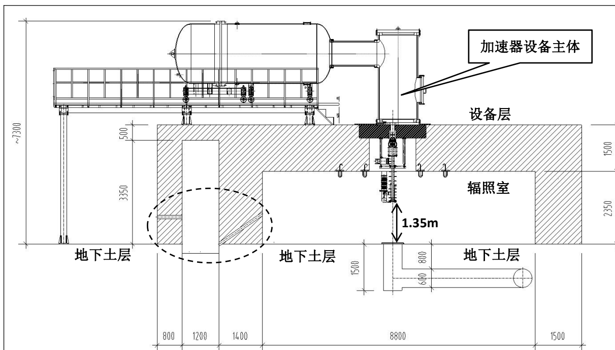
图 10-4 辐照室东南-西北方向剖面设计图
