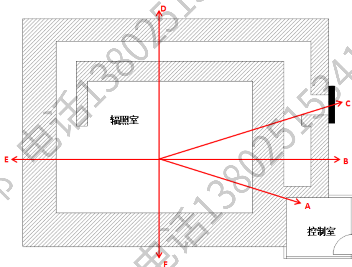
图 11-2 辐照室平面目标关注点
