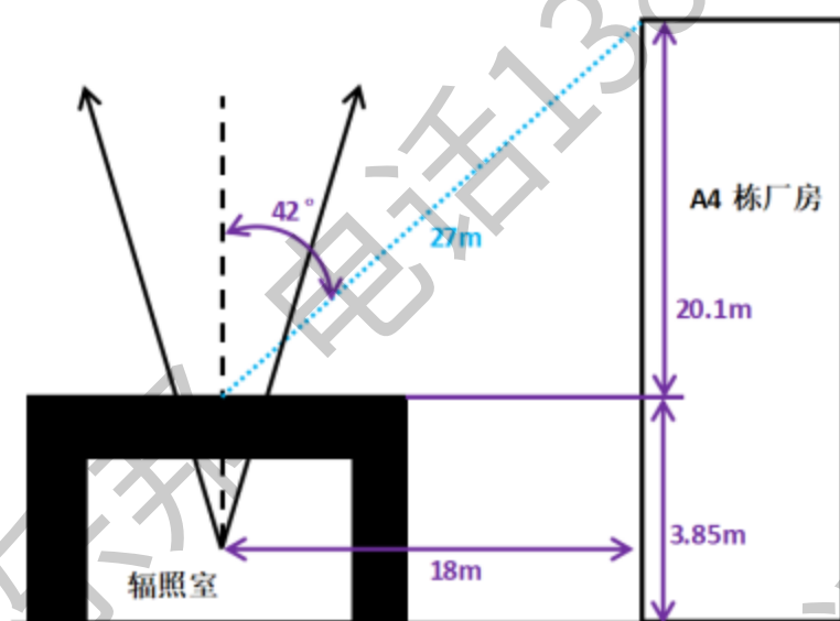
图 11-10 X 射线通过屋顶的侧向散射对 A4 栋厂房的影响示意图
