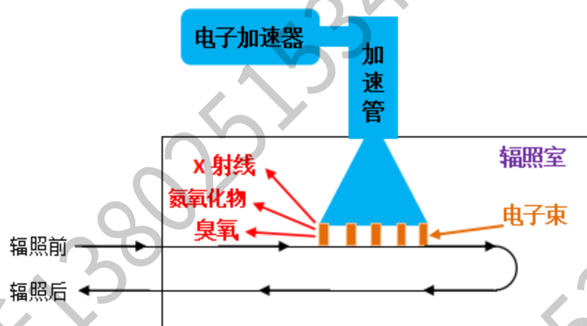
图 9-6 使用电子加速器的电子束进行辐照交联的主要产污环节示意图
