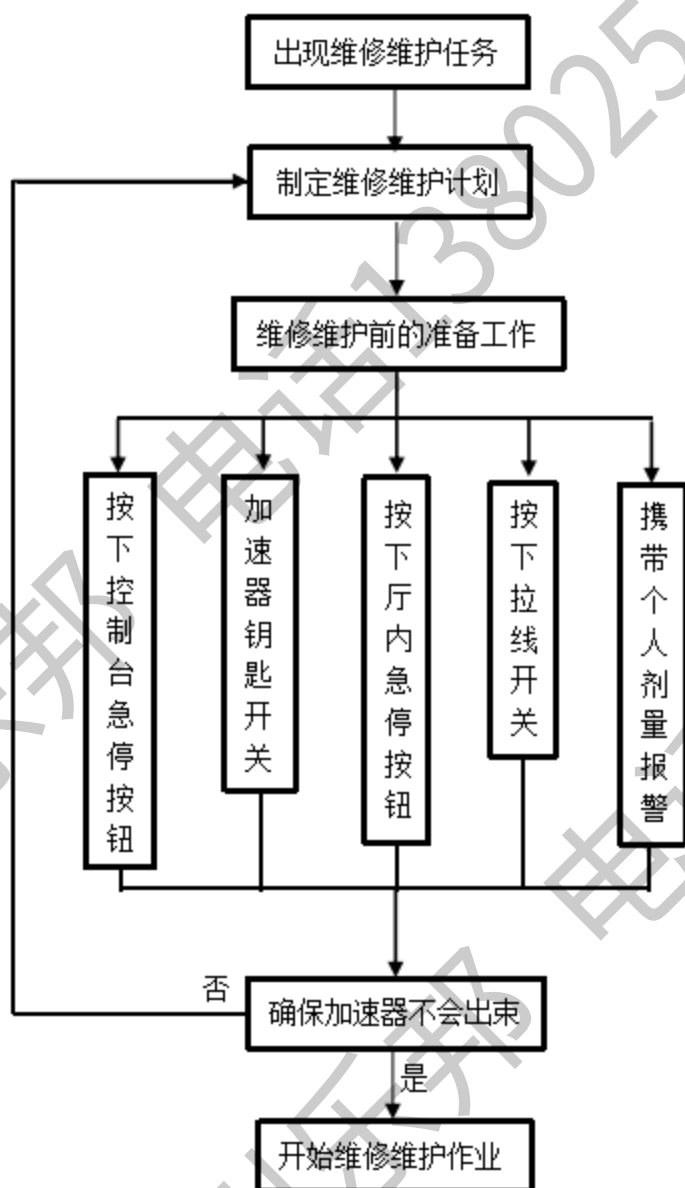
图 10-16 加速器维修维护流程图
