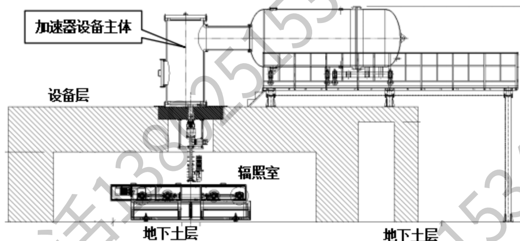
图 9-4 DDLH2.0/50-1600 型电子加速器整体结构示意图
