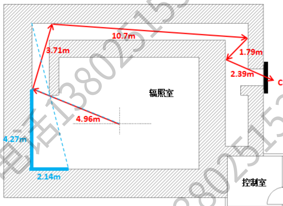
图 11-4 辐照室迷路散射路径
