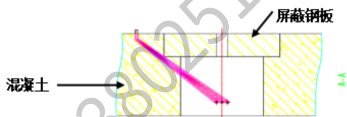
图 10-10-1 电缆沟穿过屏蔽墙的设计图（剖面图）
