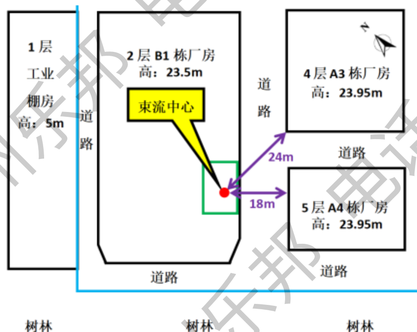
图 11-8 辐照室束流中心与 A3 和 A4 栋厂房的水平距离
