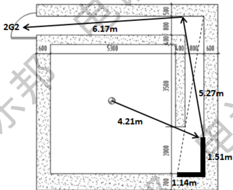
图 11-7 主机室迷路散射路径
