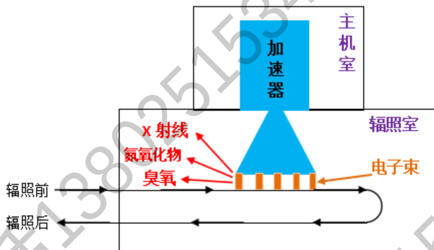
图 9-3 使用电子加速器的电子束进行辐照交联的主要产污环节示意图
