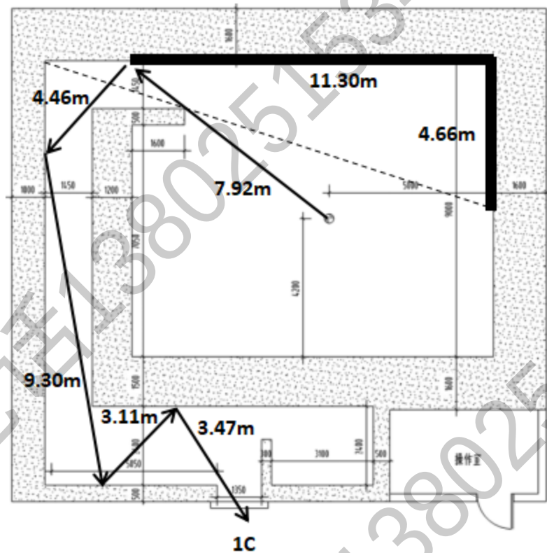
图 11-6 辐照室迷路散射路径
