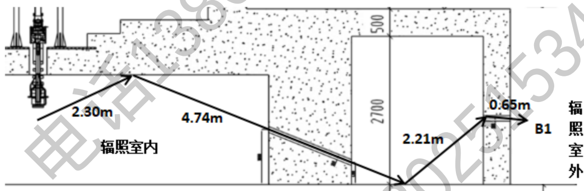
图 11-12 辐照材料进出孔的散射路径
