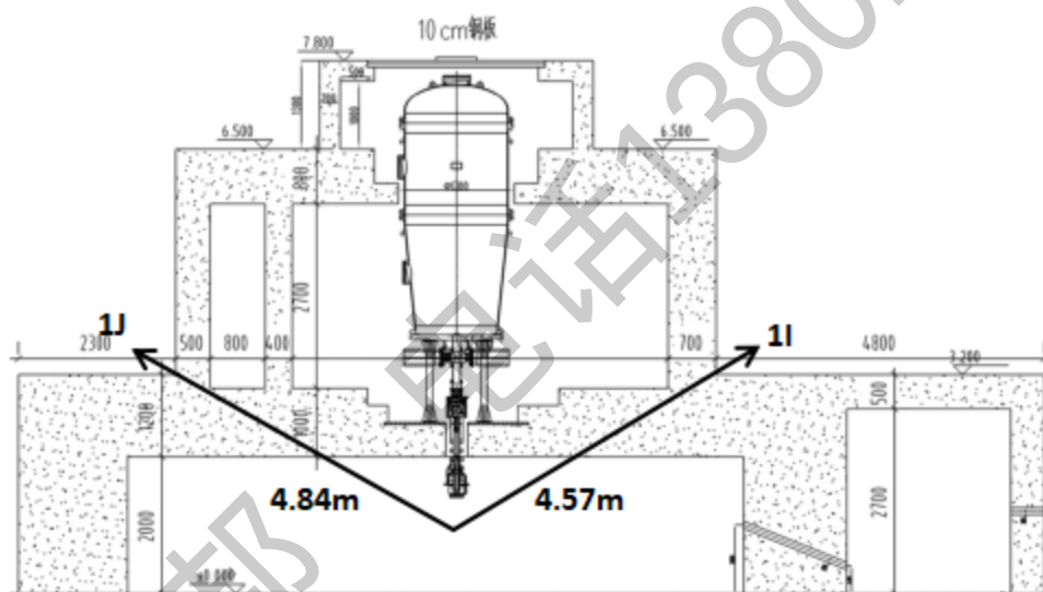
图 11-4 辐照室目标关注点（剖面图）
