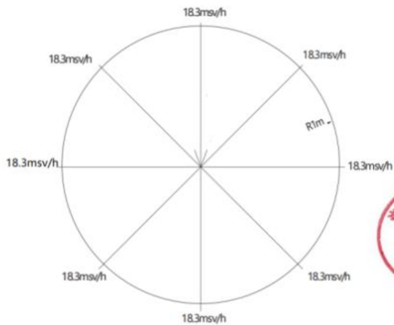
XXGH-3005Z 型 X 射线探伤机
