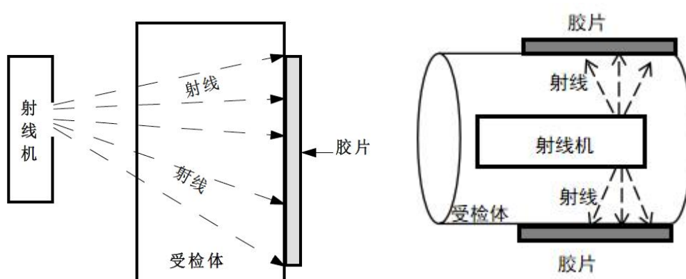
图 9-2 探伤工作原理图
