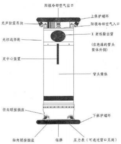
图3: 定向管头
