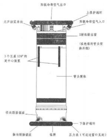
图2: 周向径射束管头
