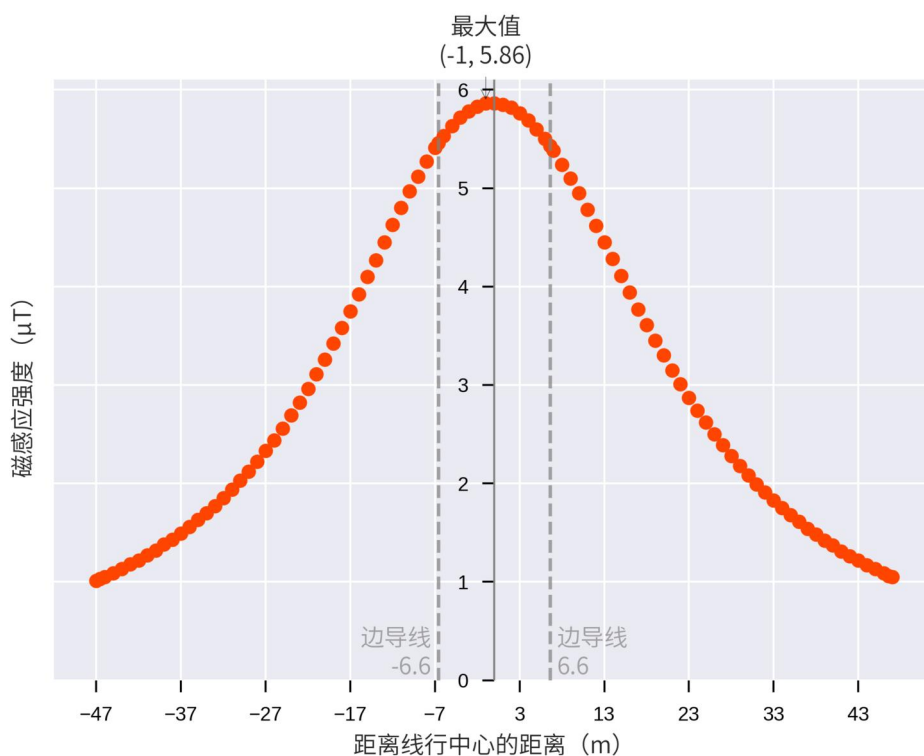
图 7 新建 220kV 丽晶至五和牵引站单回线路工程（架空段）工频磁场预测结果分布图（地面 1.5m 处）
