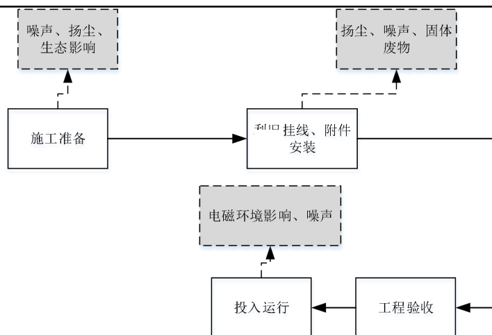
图3 新建架空线路工程施工工序流程及产污示意图
