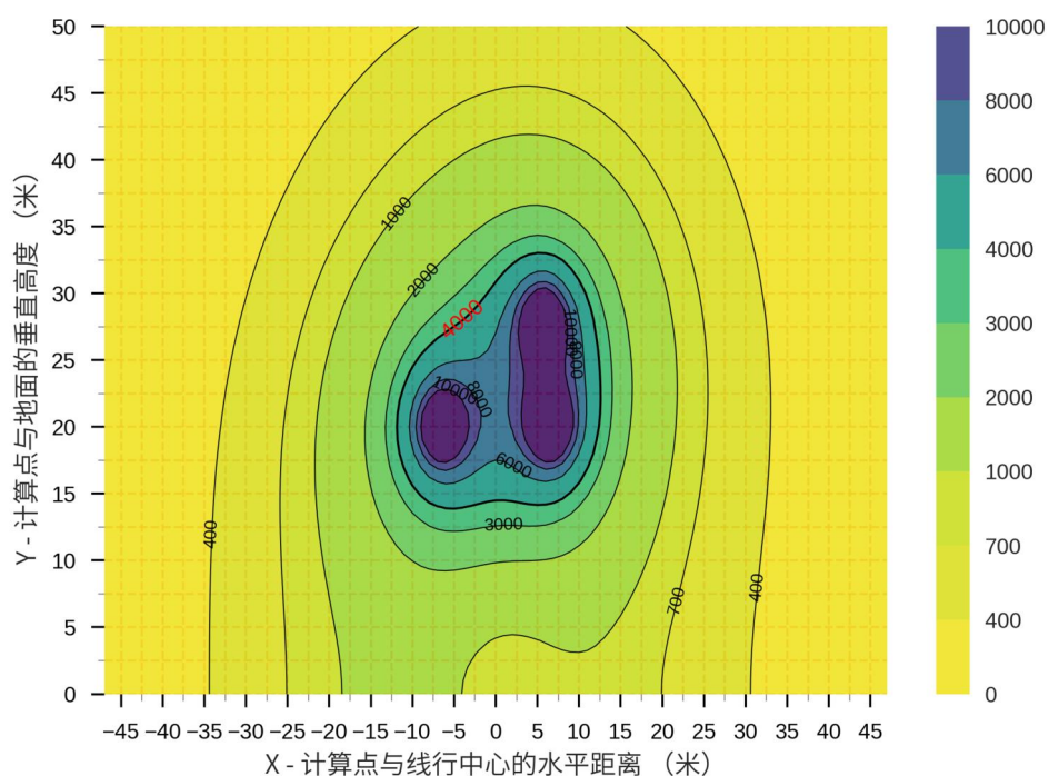
图 6 新建 220kV 丽晶至五和牵引站单回线路工程（架空段）工频电场预测结果等值线图
