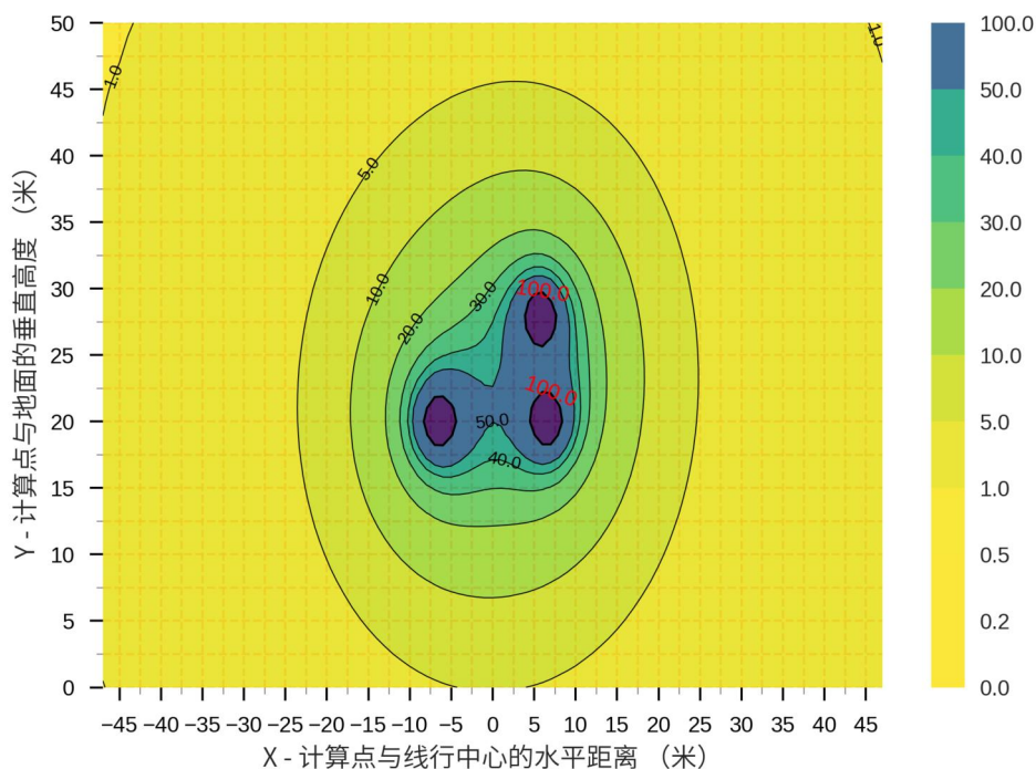
图8 新建220kV 丽晶至五和牵引站单回线路工程（架空段）工频磁场预测结果等值线图
