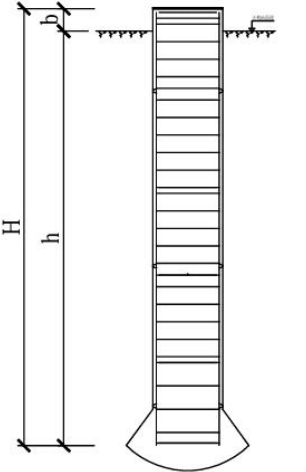
人工挖孔桩基础
