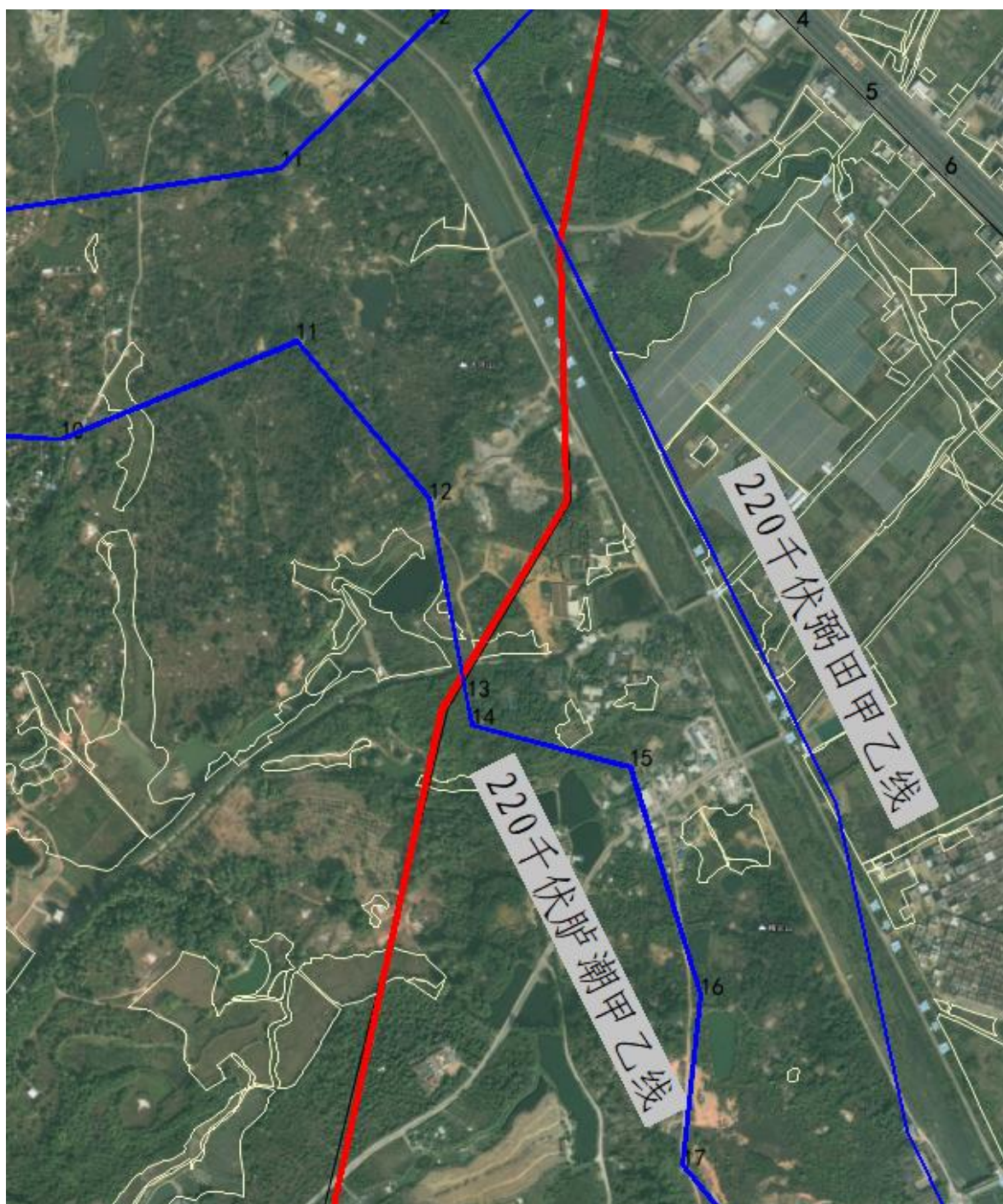
图 7.4.5 拟建线路穿越现有 220kV 线路
