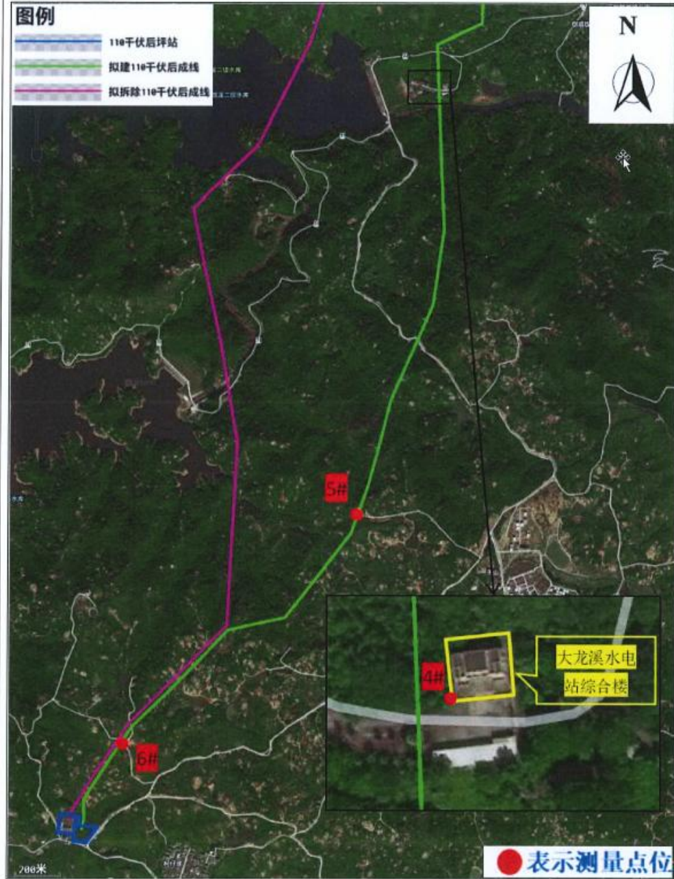
图2 本工程检测布点示意图 2
