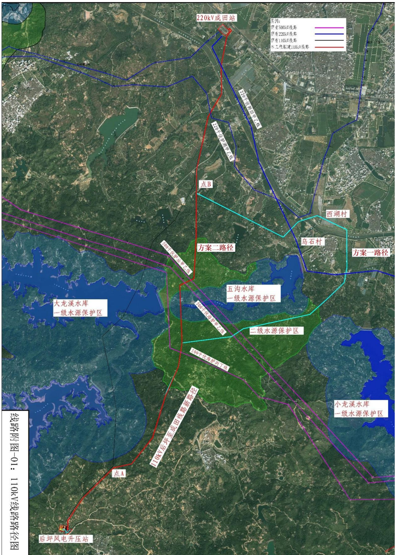
图 7.1.1 110kV 线路路径比选方案示意图
