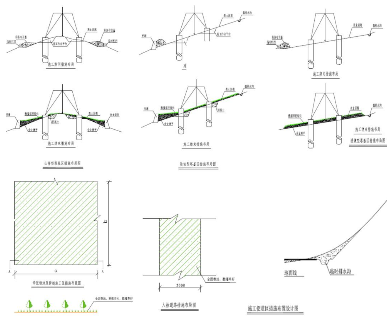
附图 15 典型生态环境保护措施设计图
