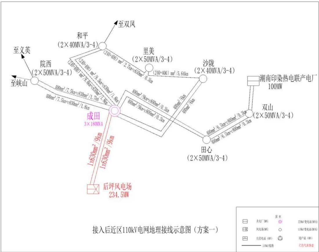
接入系统示意图
