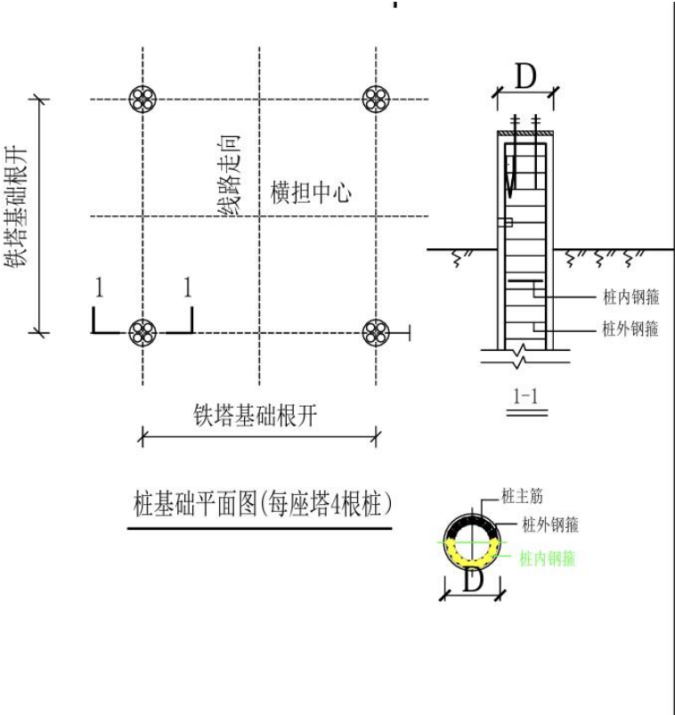
人工挖孔桩基础
