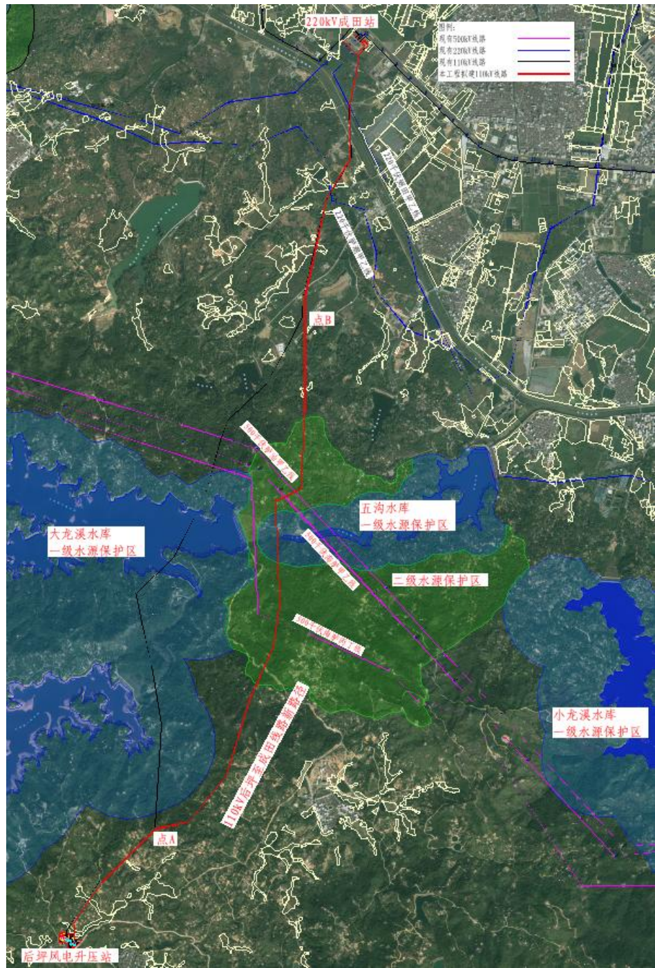
图 7.4.4 方案二线路路径方案图
